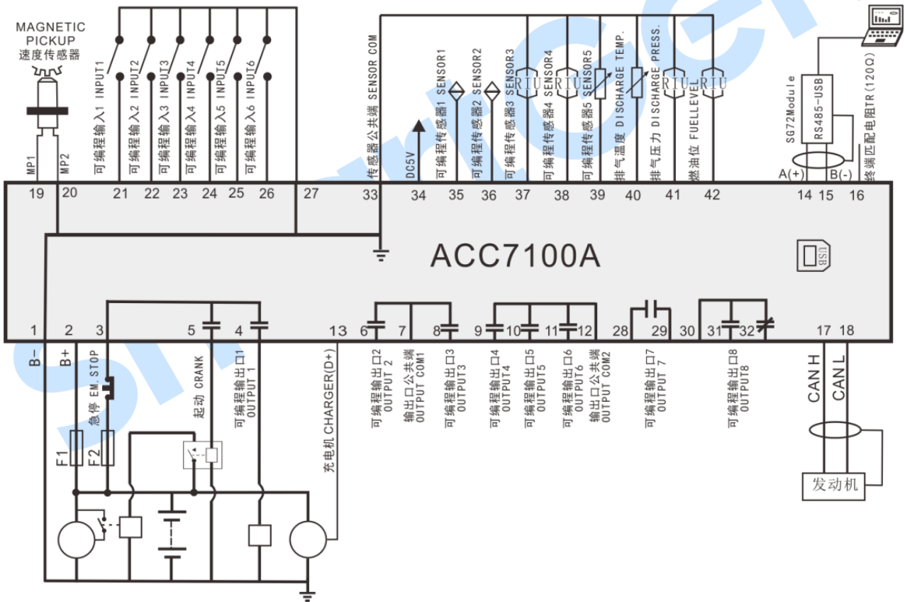
图8 ACC7100A 典型应用图
