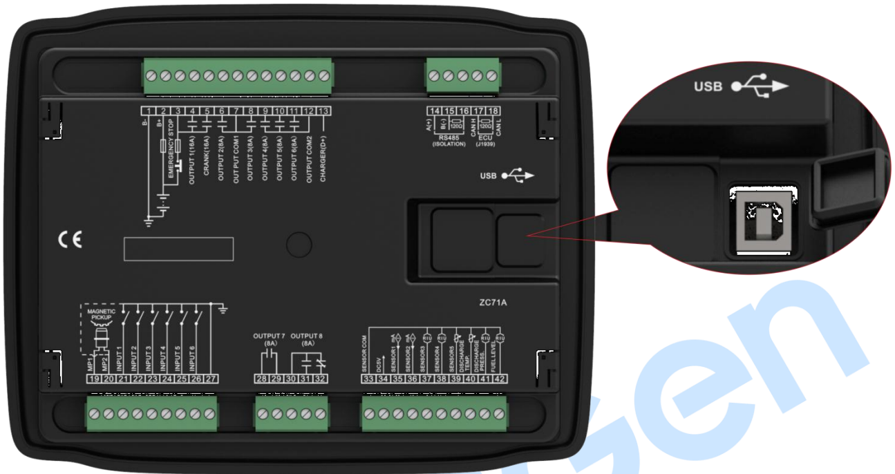
图6 控制器背面板图
