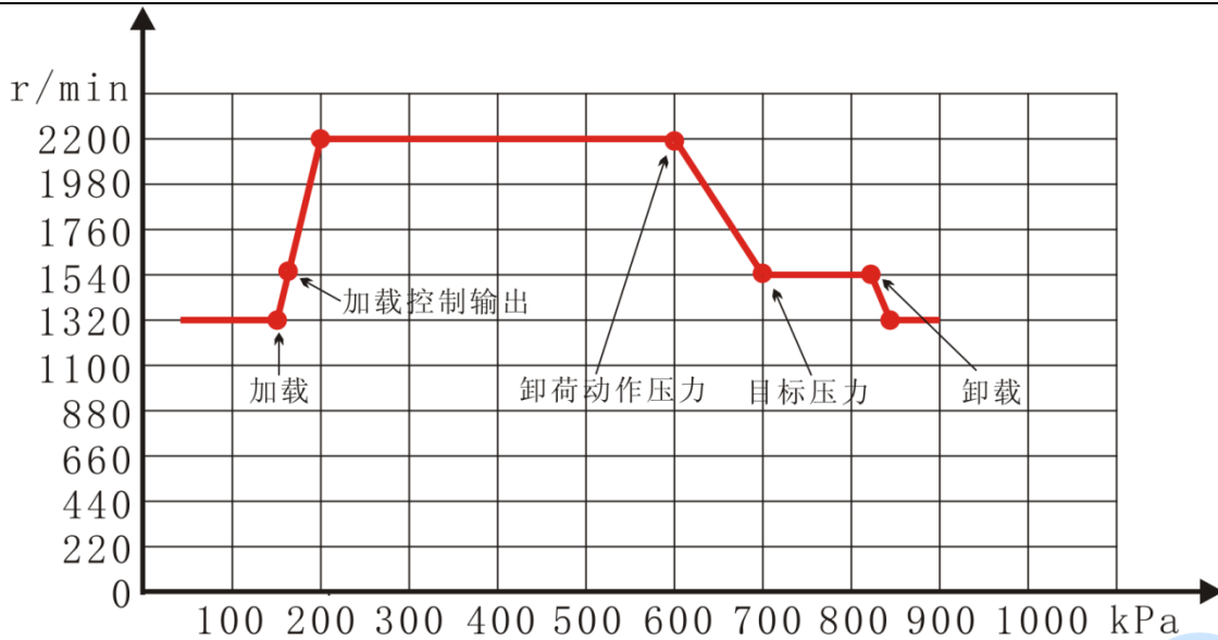
图2 转速-排气压力曲线图
