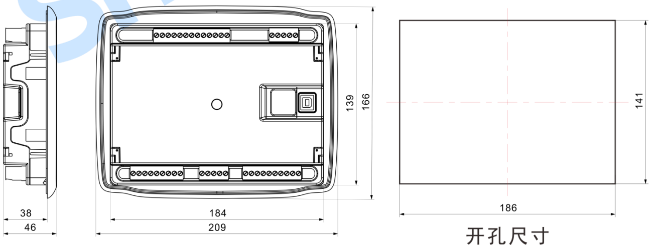
图10 外形及开孔尺寸
