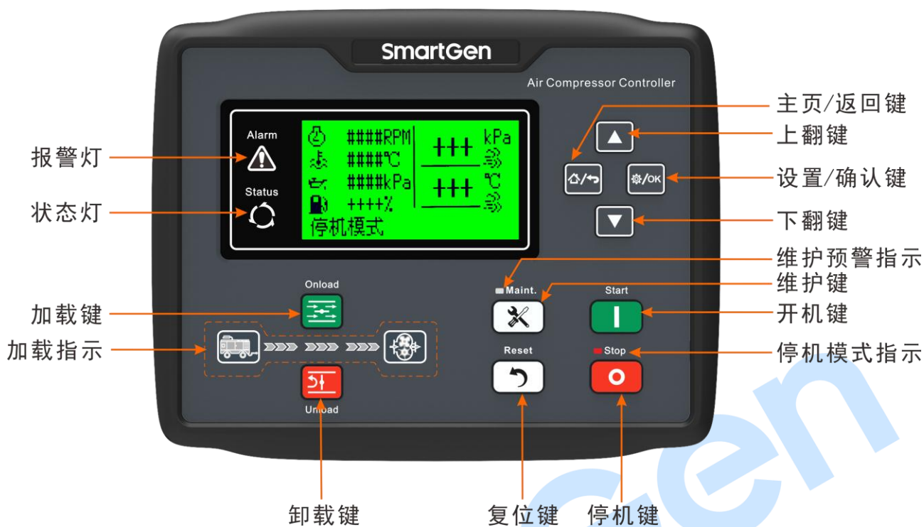
图1 前面板图
