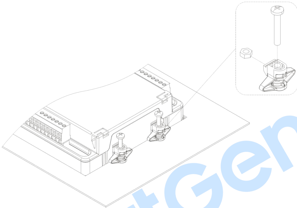
图9 ACC7100A 卡件安装示意图
