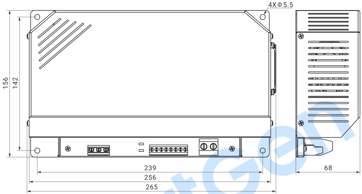
图6 BACM2420A 安装尺寸图
