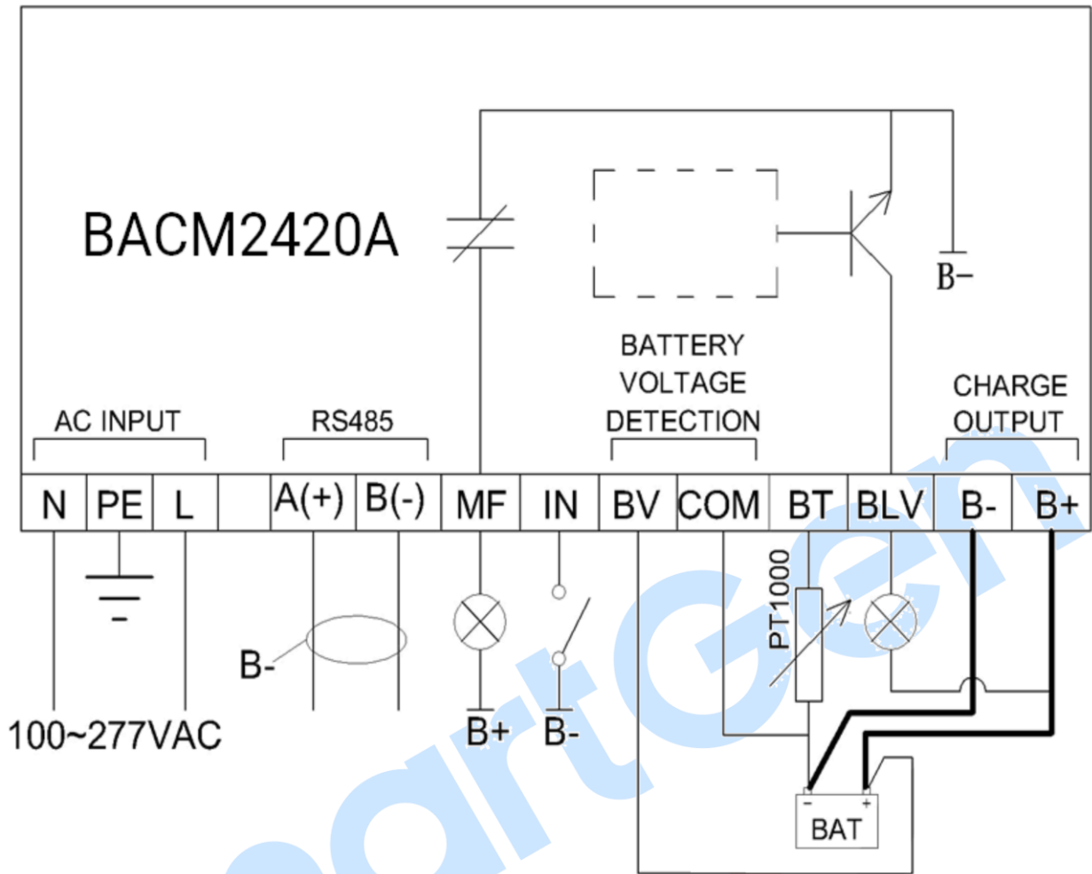
图5 接线图
