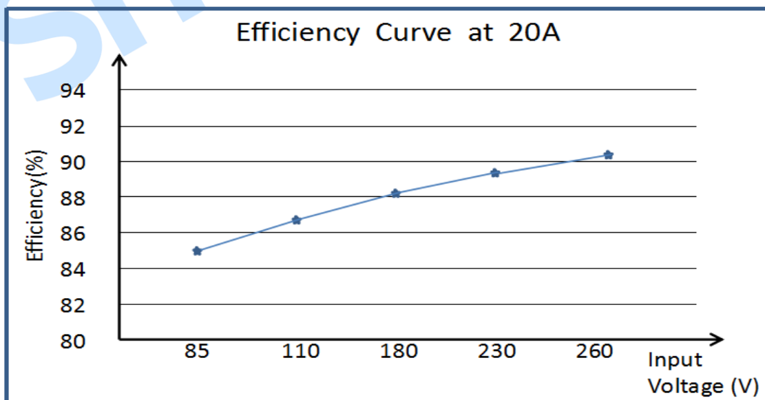
图3 效率曲线
