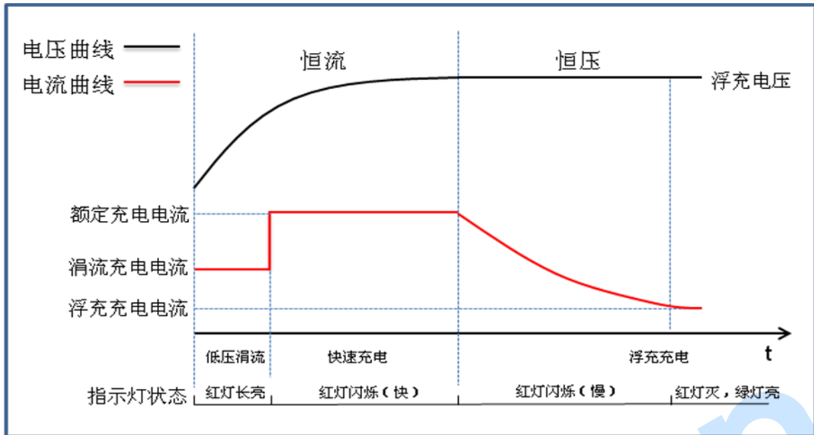
图2 二段式充电曲线图
