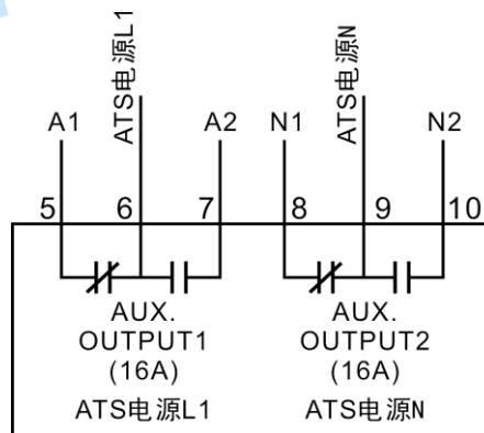
图9 ATS 电源相电压供电
