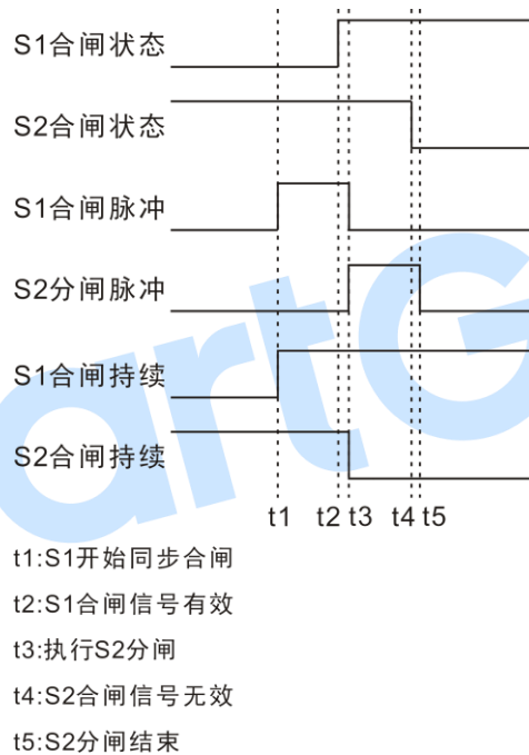
图7 S1 同步合闸过程波形图
