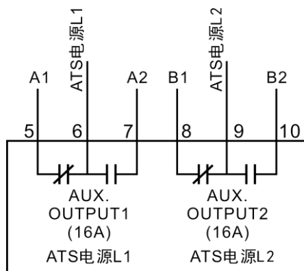
图10 ATS 电源线电压供电
