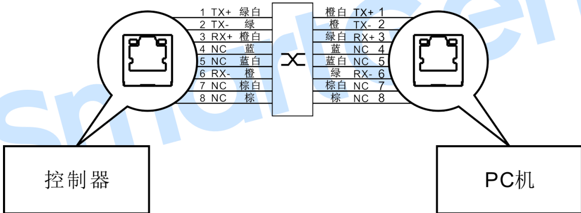
图14 控制器与 PC 机交叉线连接示意图
