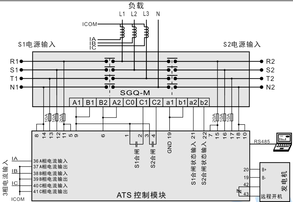
图20 SGQ-M 应用图
