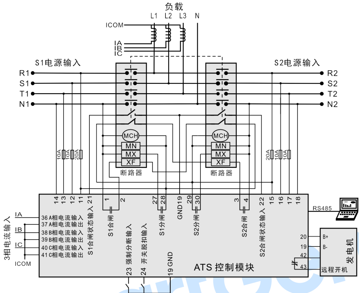
图24 断路器应用图
