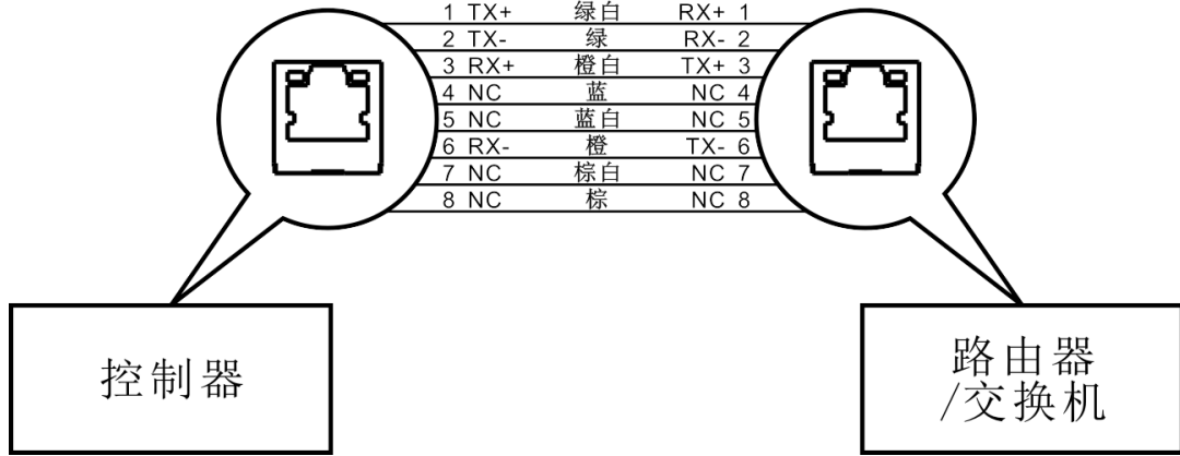
图13 控制器与路由器直连示意图
