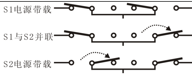
图6 同步切换示意图
