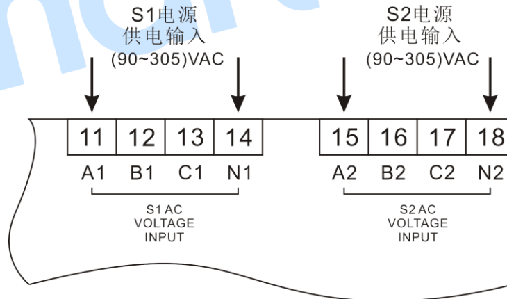
图17 交流供电示意图
