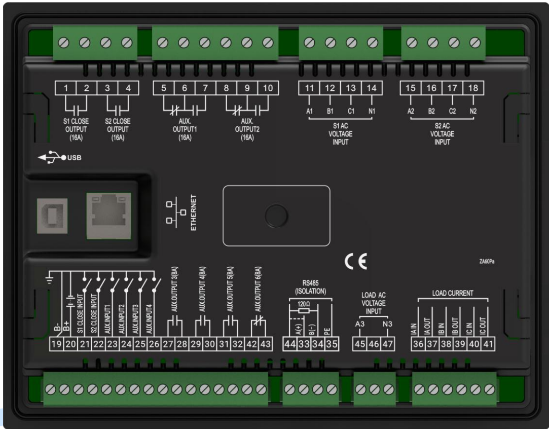
图15 控制器后面板图
