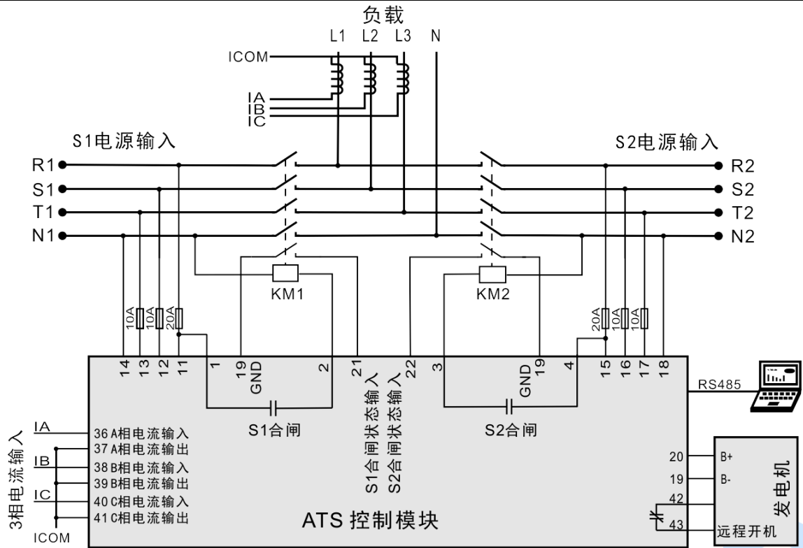
图23 接触器应用图
