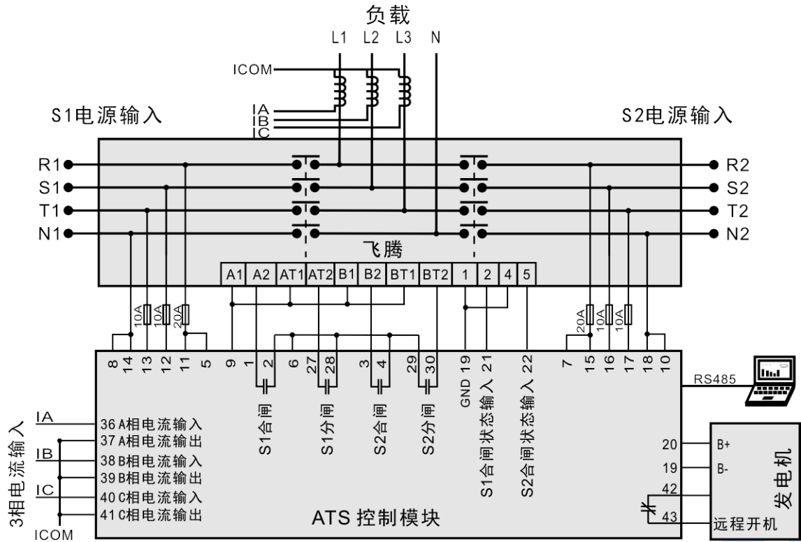
图22 飞腾应用图
