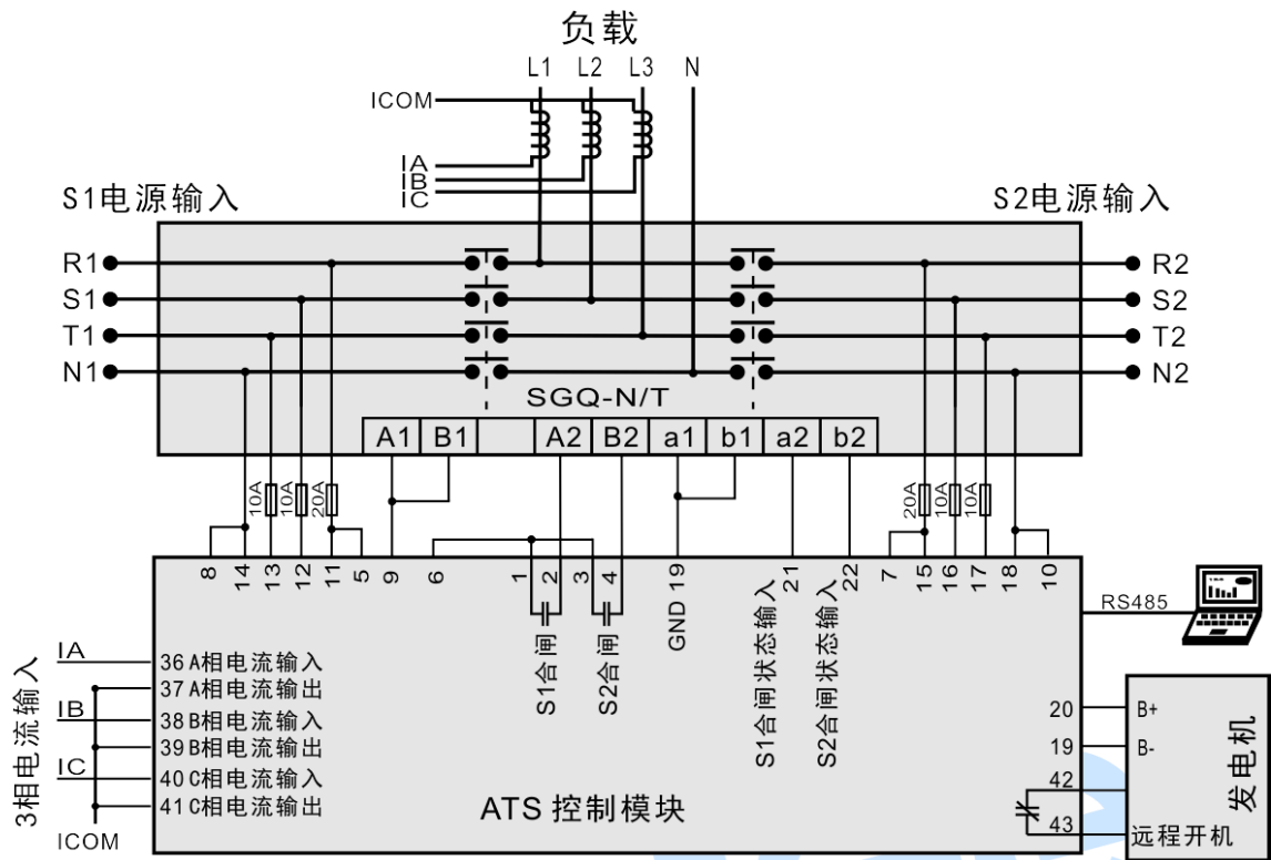
图19 SGQ-N/T 应用图
