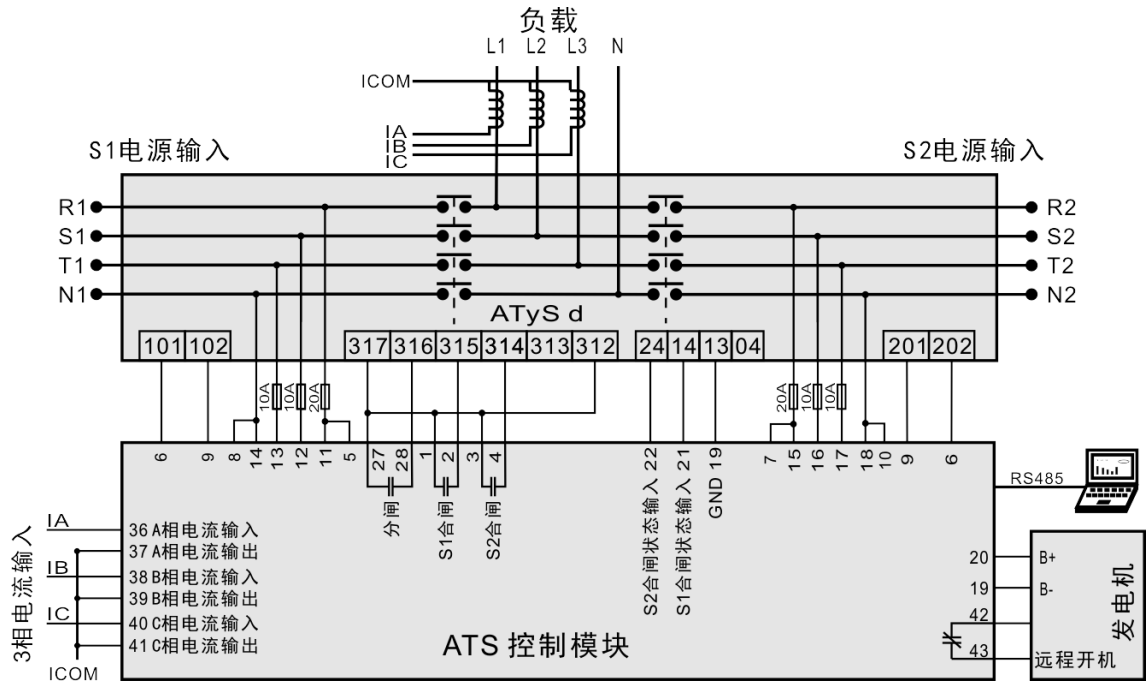
图21 ATyS d 应用图
