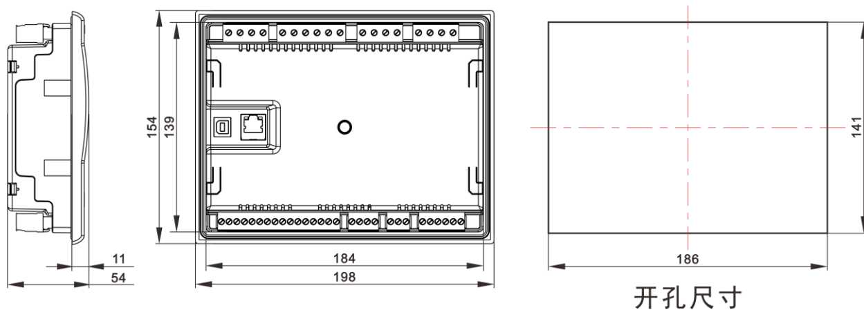
图25 外形尺寸及面板开孔尺寸
