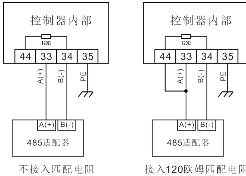
图18 RS485 连接示意图
