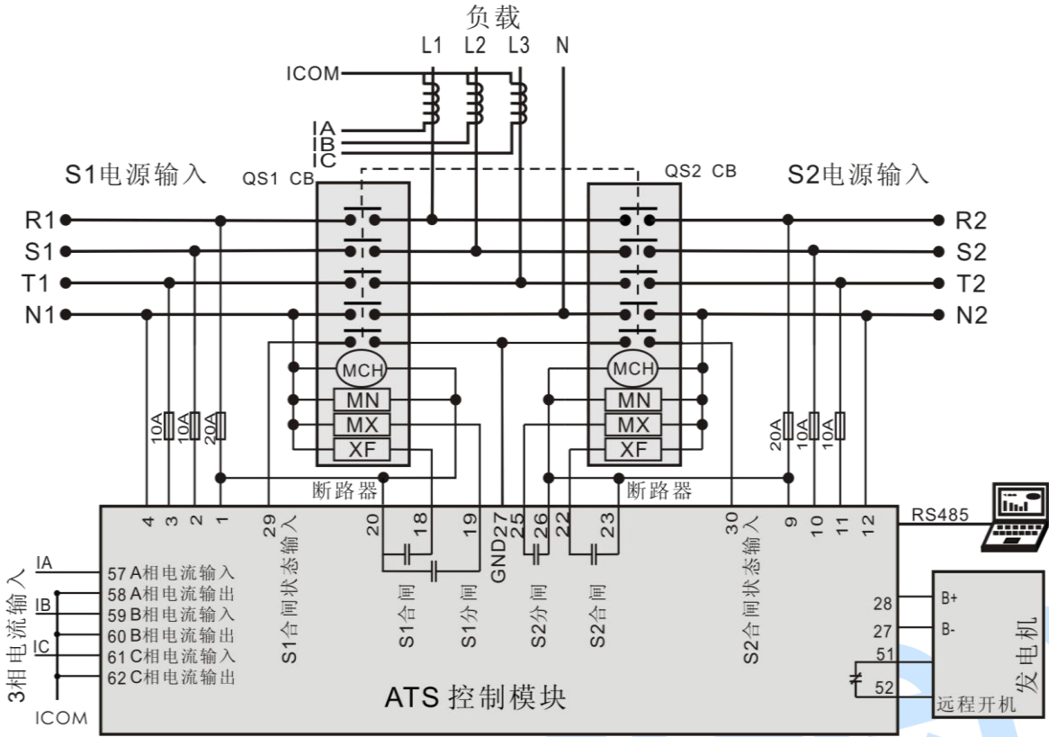
图15 断路器应用图
