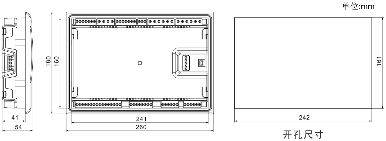
图16 外形尺寸及面板开孔尺寸
