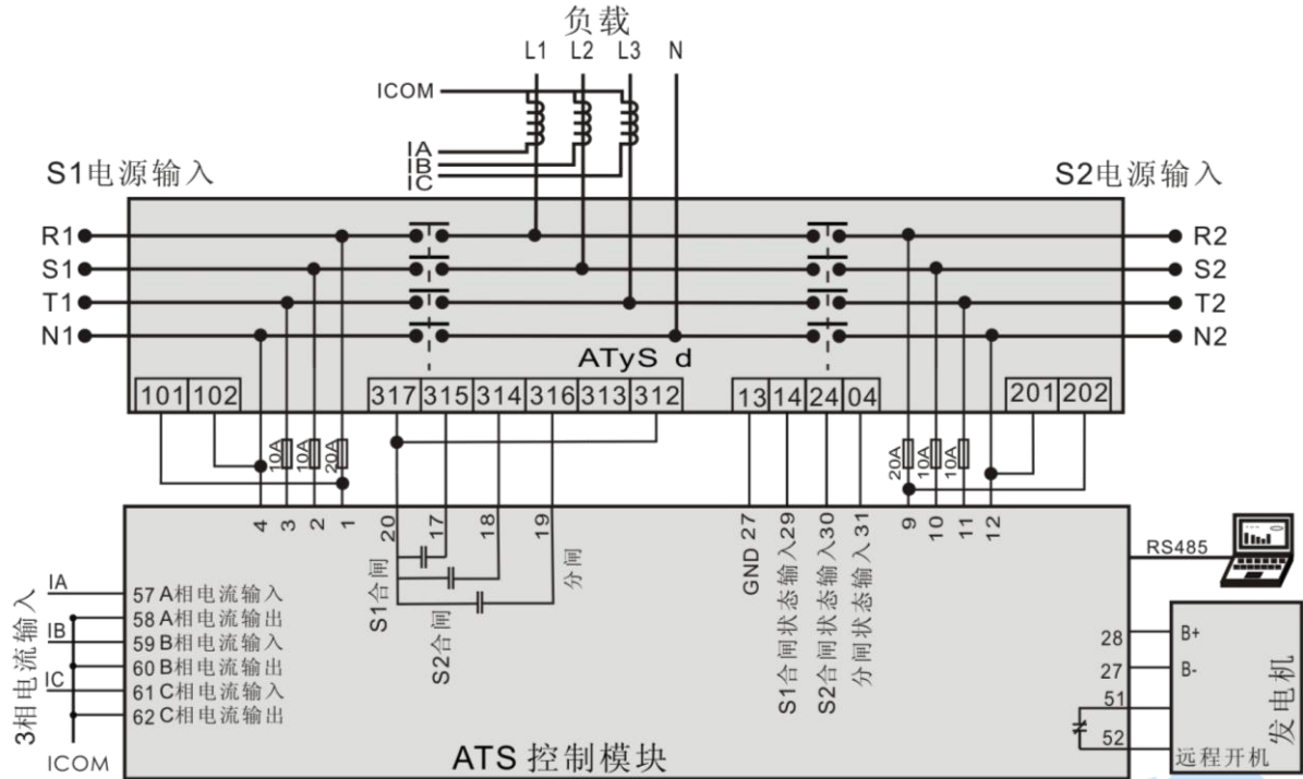
图12 ATyS d 应用图
