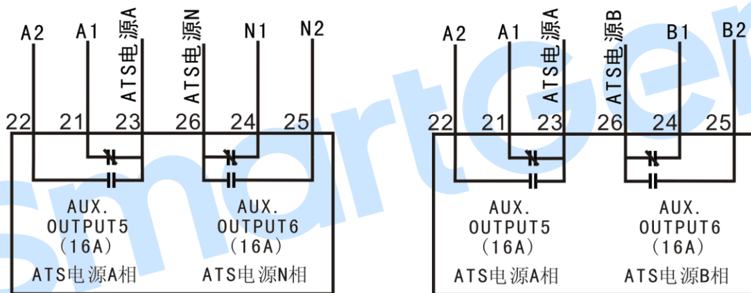
图5 ATS 电源相电压供电和线电压供电连接图示
