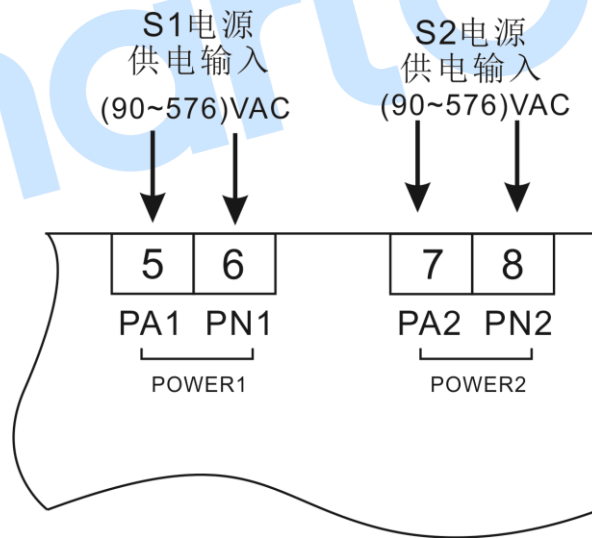
图8 交流供电示意图
