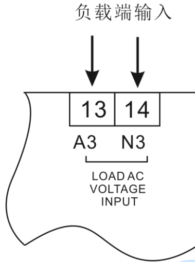
图9 负载有电检测接线示意图
