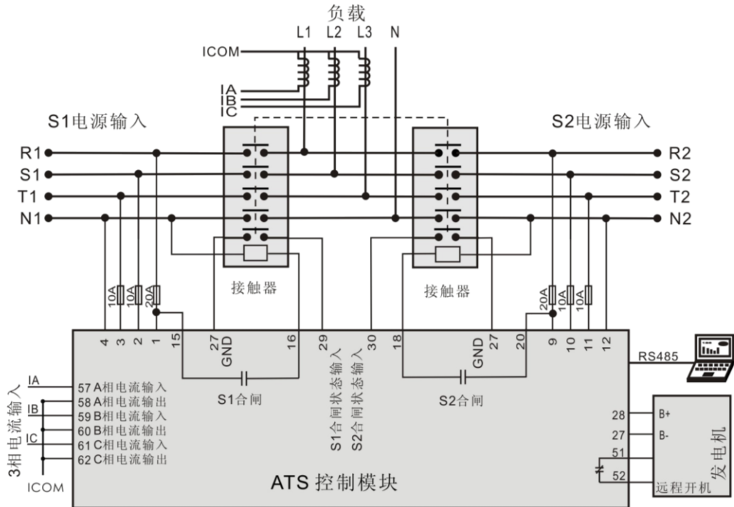
图14 接触器应用图
