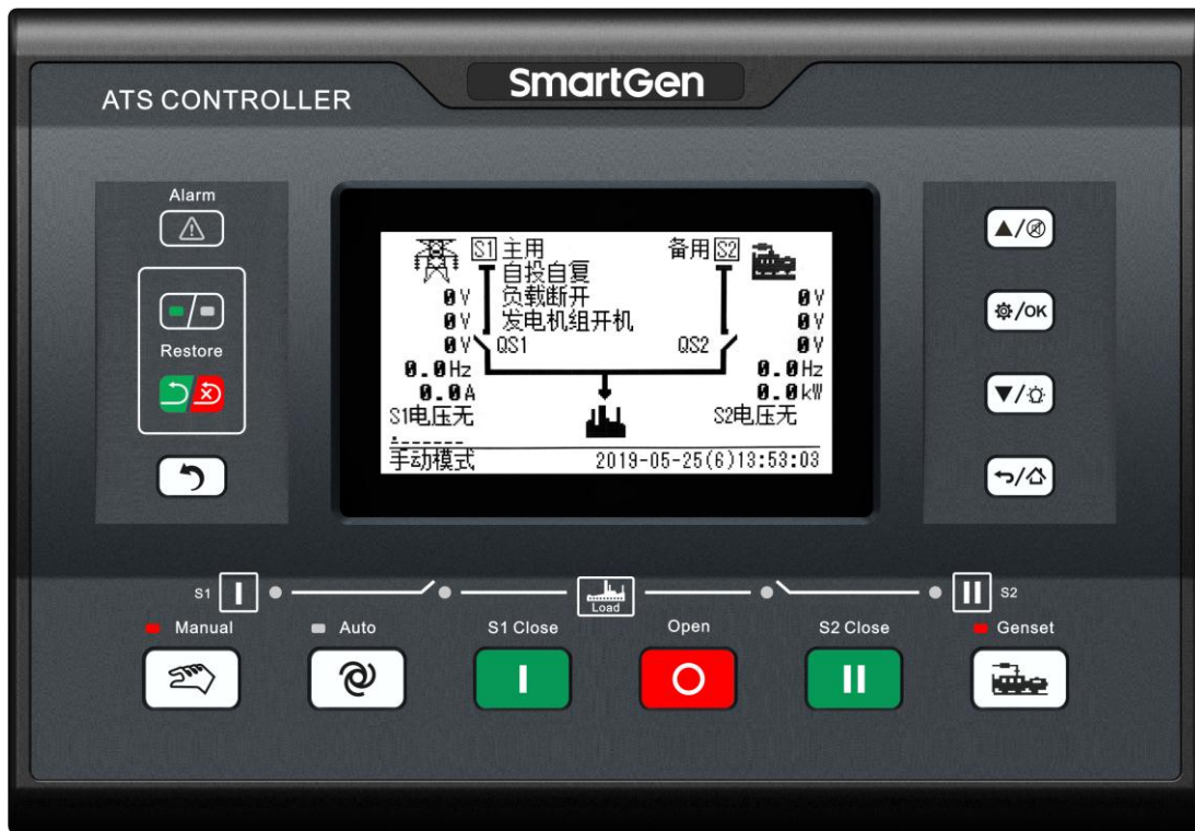
图2 面板指示图
