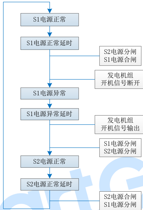
图3 自投自复流程图
