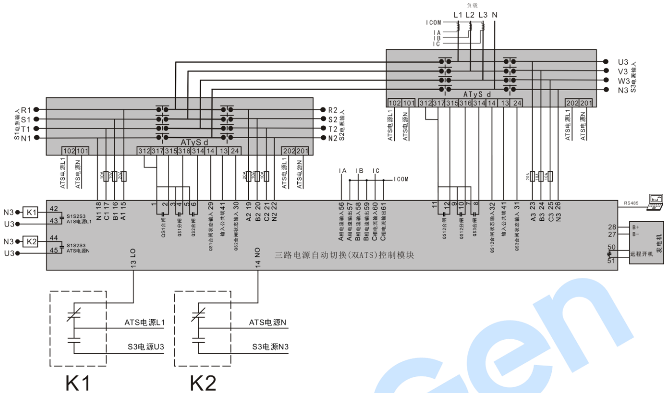
图9 ATyS d 应用图二
