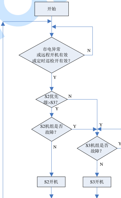
图3 主备开机流程图
