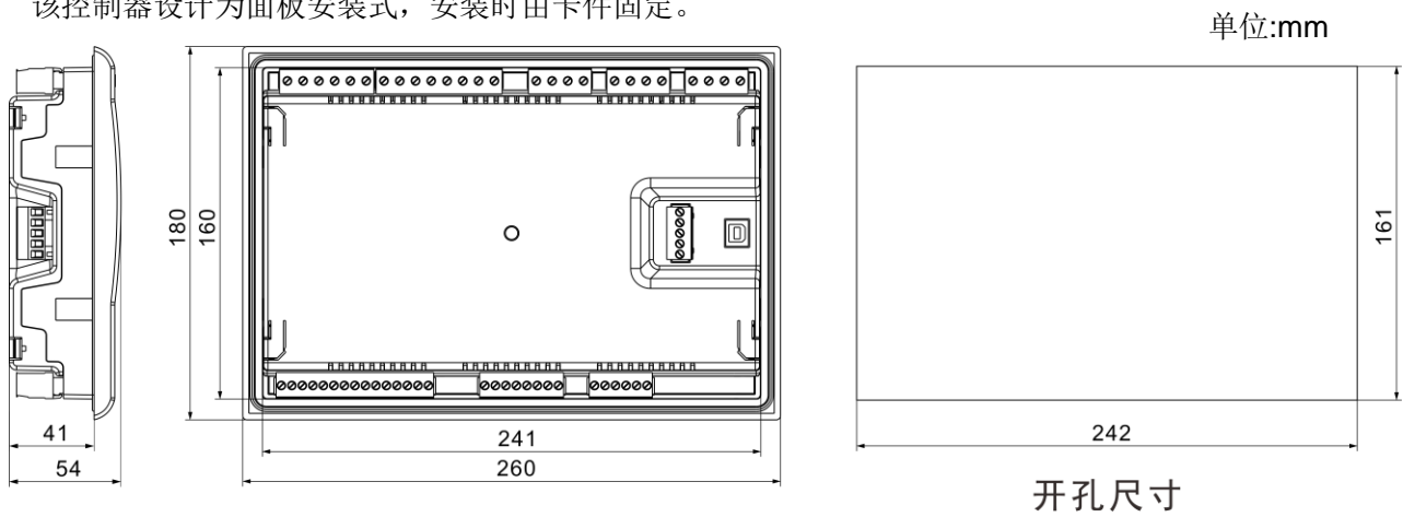
图13 外形尺寸及面板开孔尺寸
