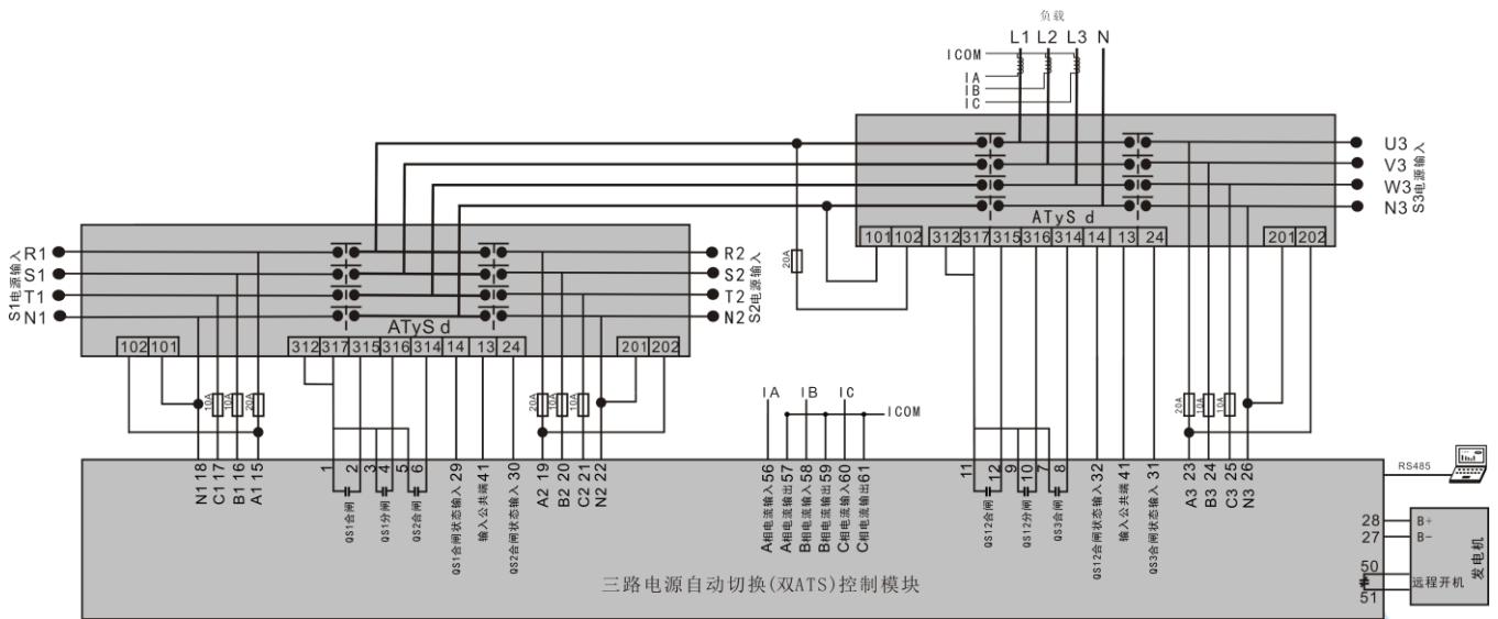
图8 ATyS d 应用图一
