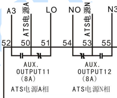
图6 ATS 电源由 S1S2S3 中任一相供电连接图示
