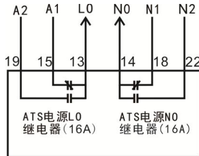
图5 ATS 电源 LO-NO 输出内部连接图示
