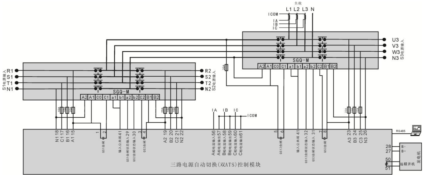
图11 SGQ-M 应用图
