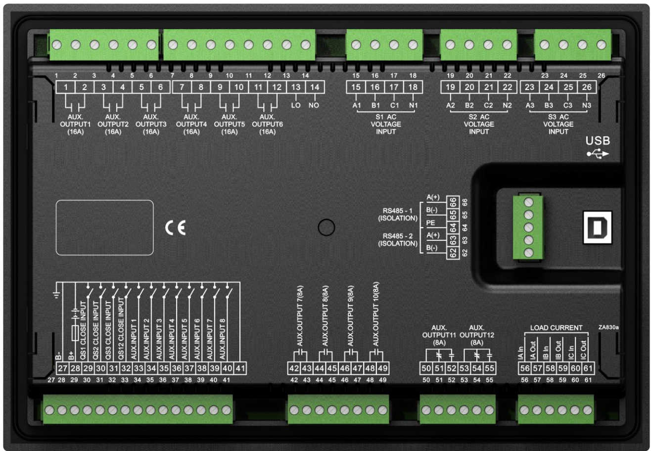
图7 控制器后面板图
