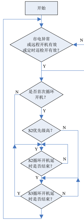
图2 循环开机流程图
