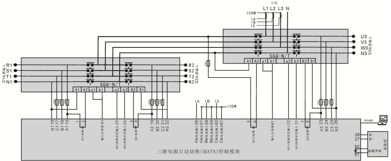
图10 SGQ-N/T 应用图
