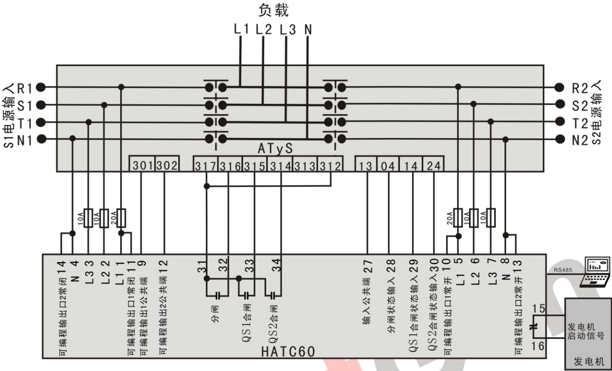
图4 开关 ATyS 应用图
