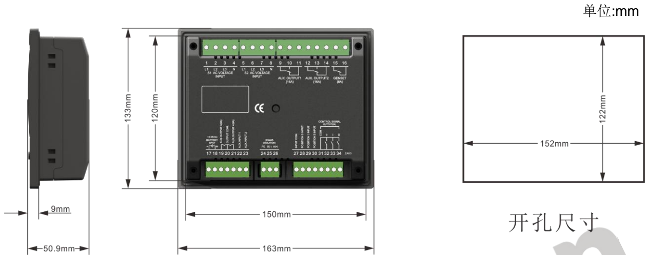
图10 外形尺寸及面板开孔尺寸
