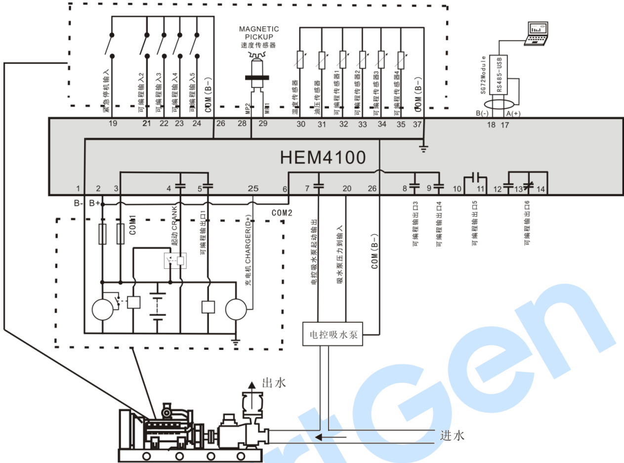
图10 接电控吸水泵的典型应用图
