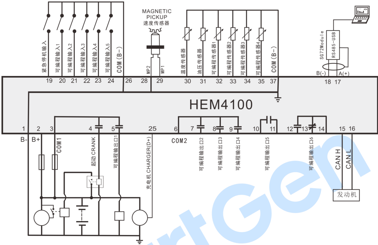
图8 HEM4100 典型应用图
