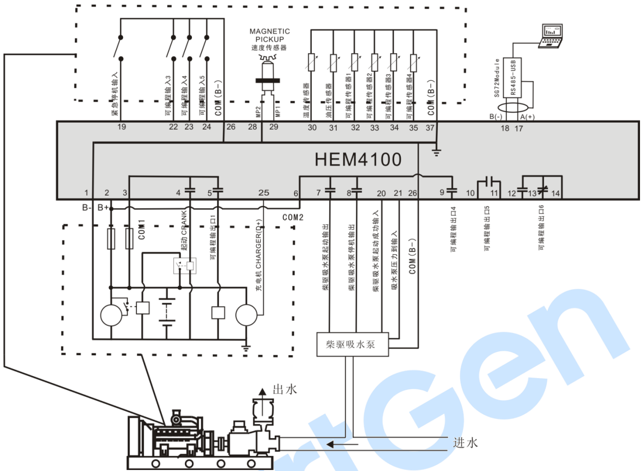
图9 接柴驱吸水泵的典型应用图
