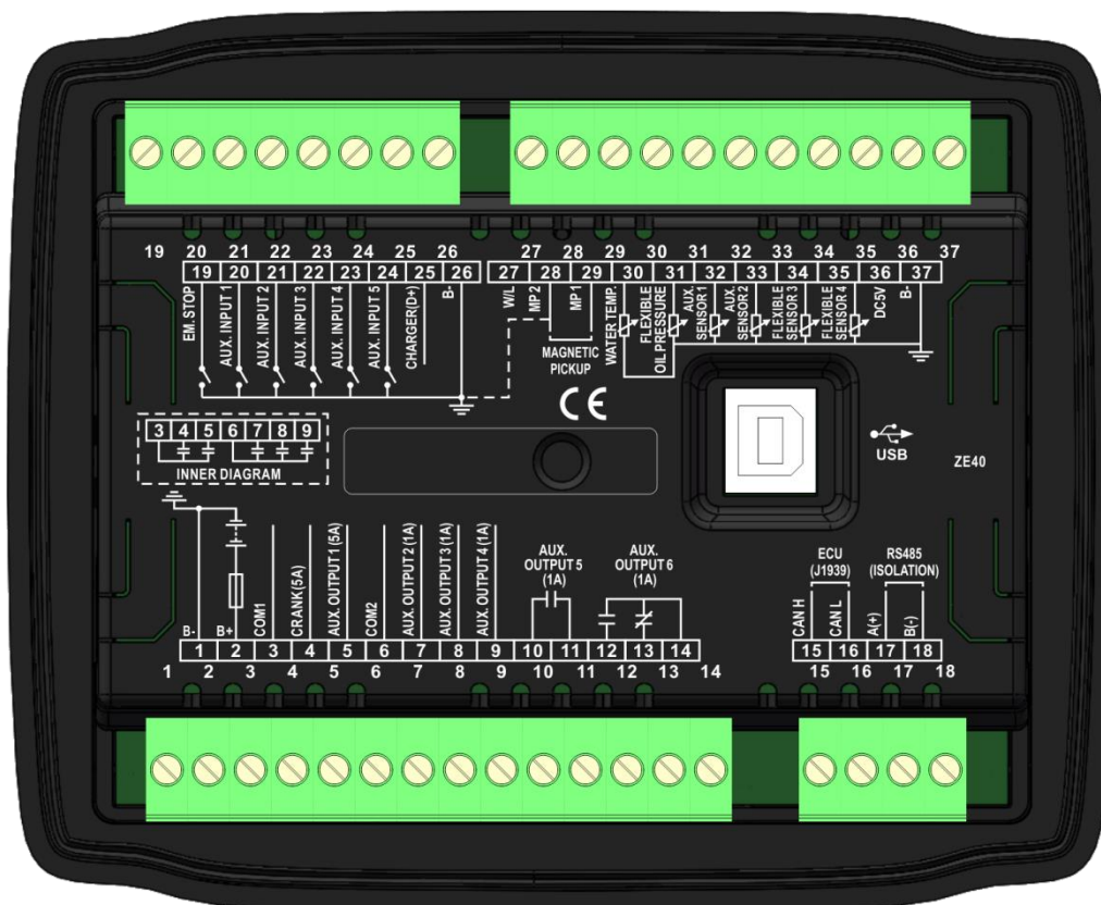
图6 控制器背面板
