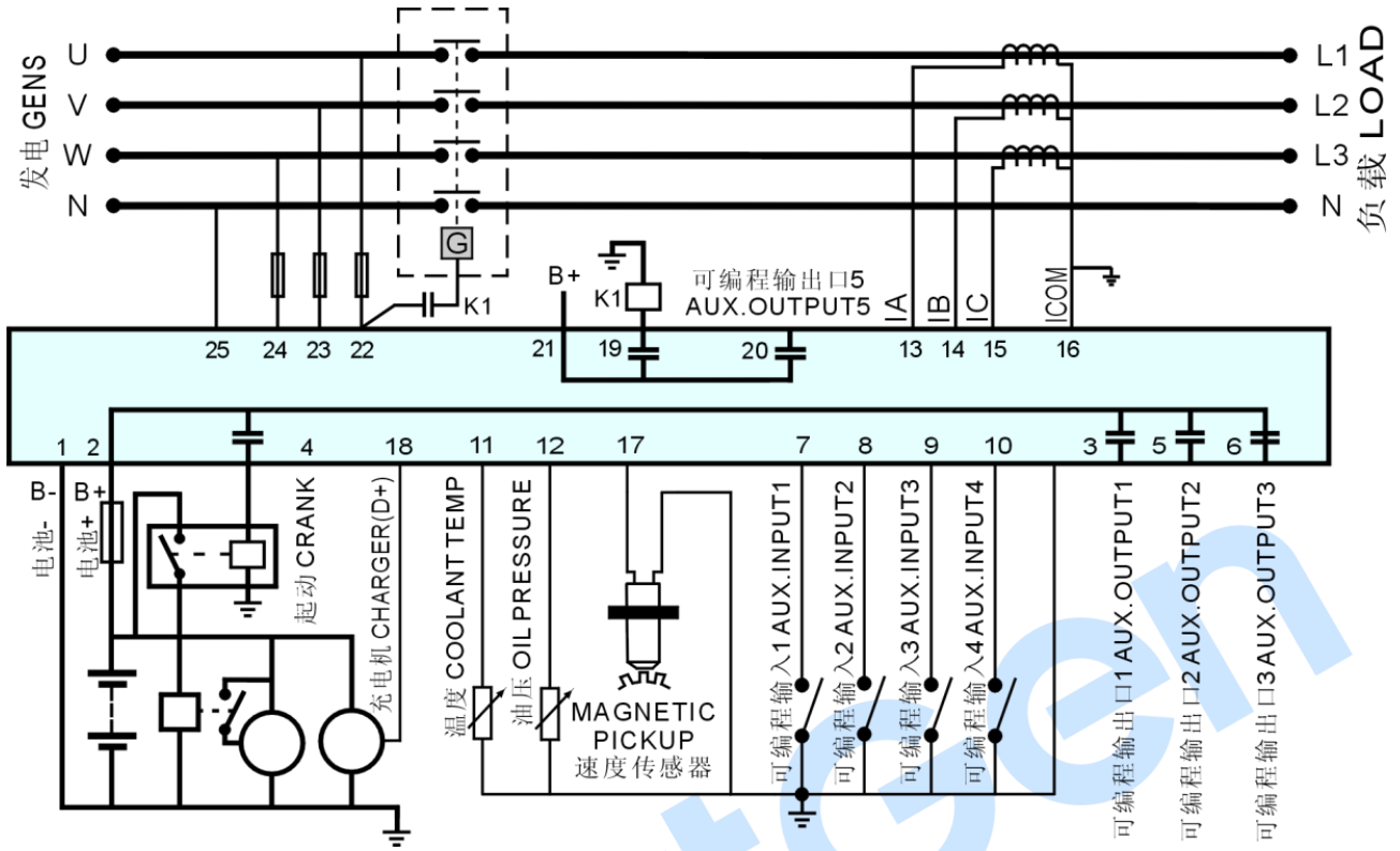
图4 HGM410N 典型应用图
