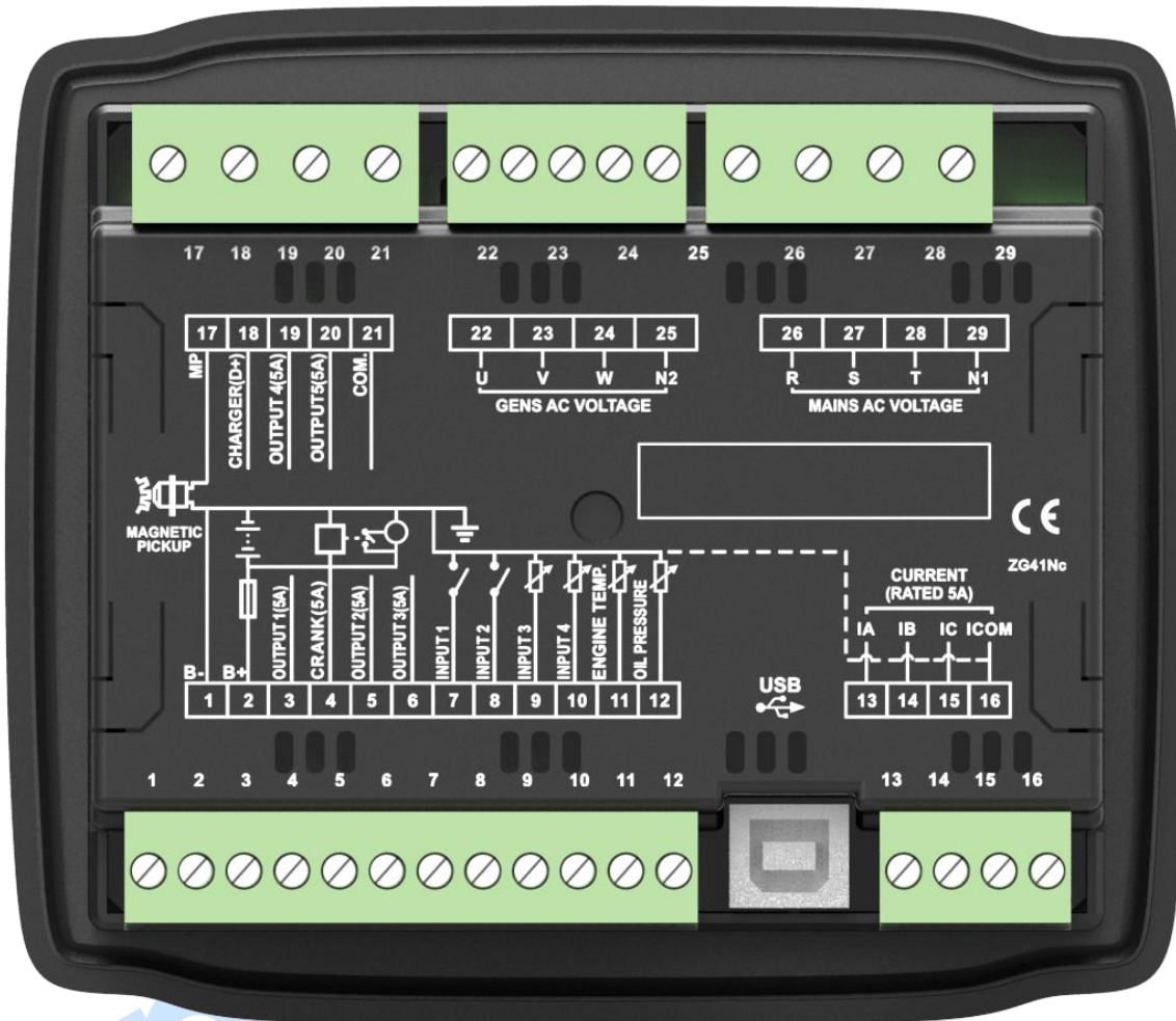
图2 控制器背面板图
