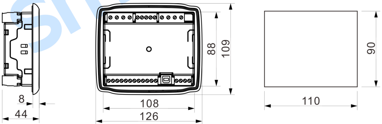
图8 外形及开孔尺寸
