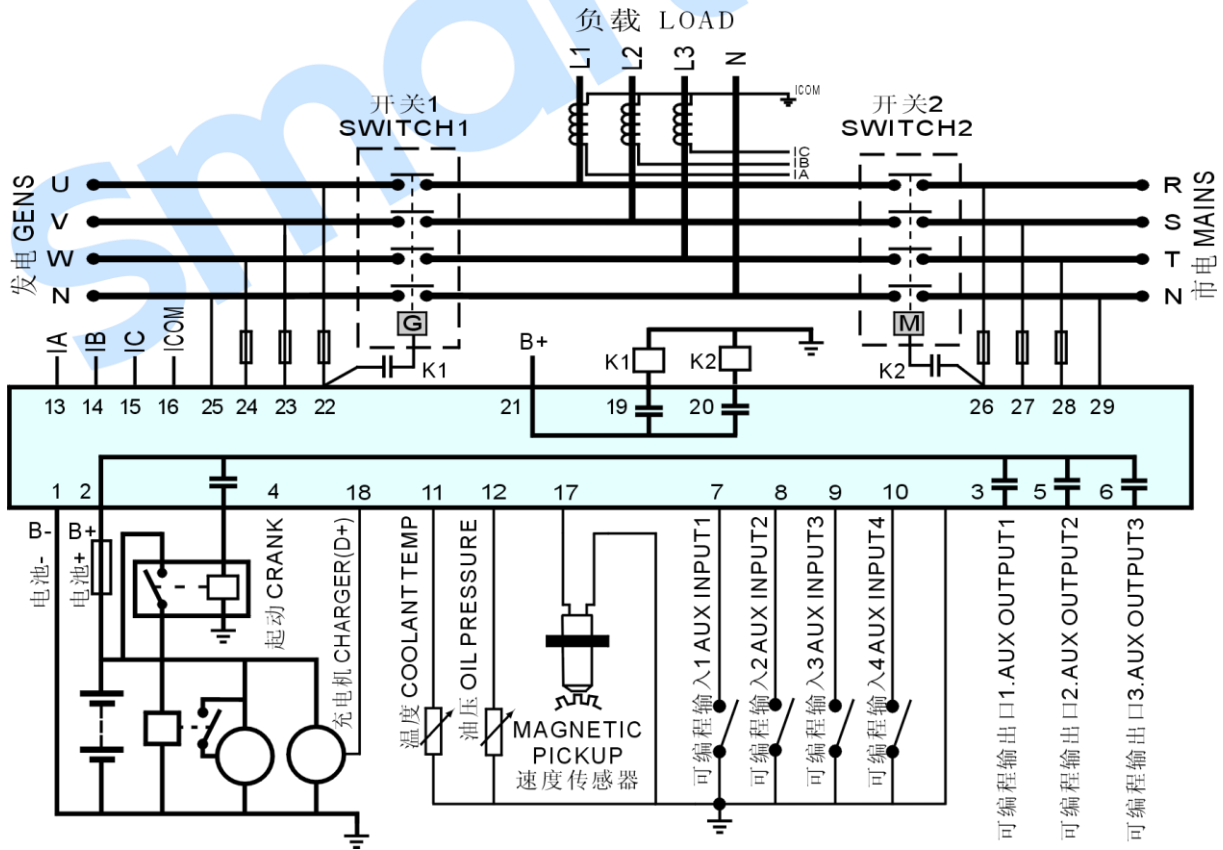
图5 HGM420N 典型应用图
