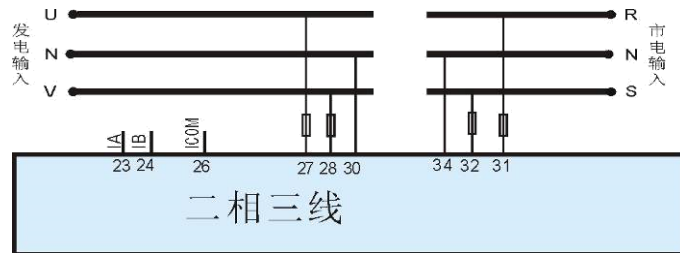
图8 二相三线接线图
