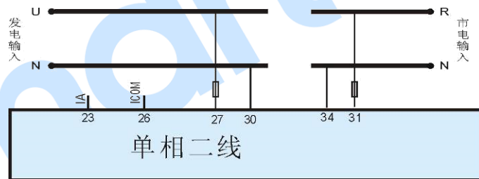
图7 单相两线接线图
