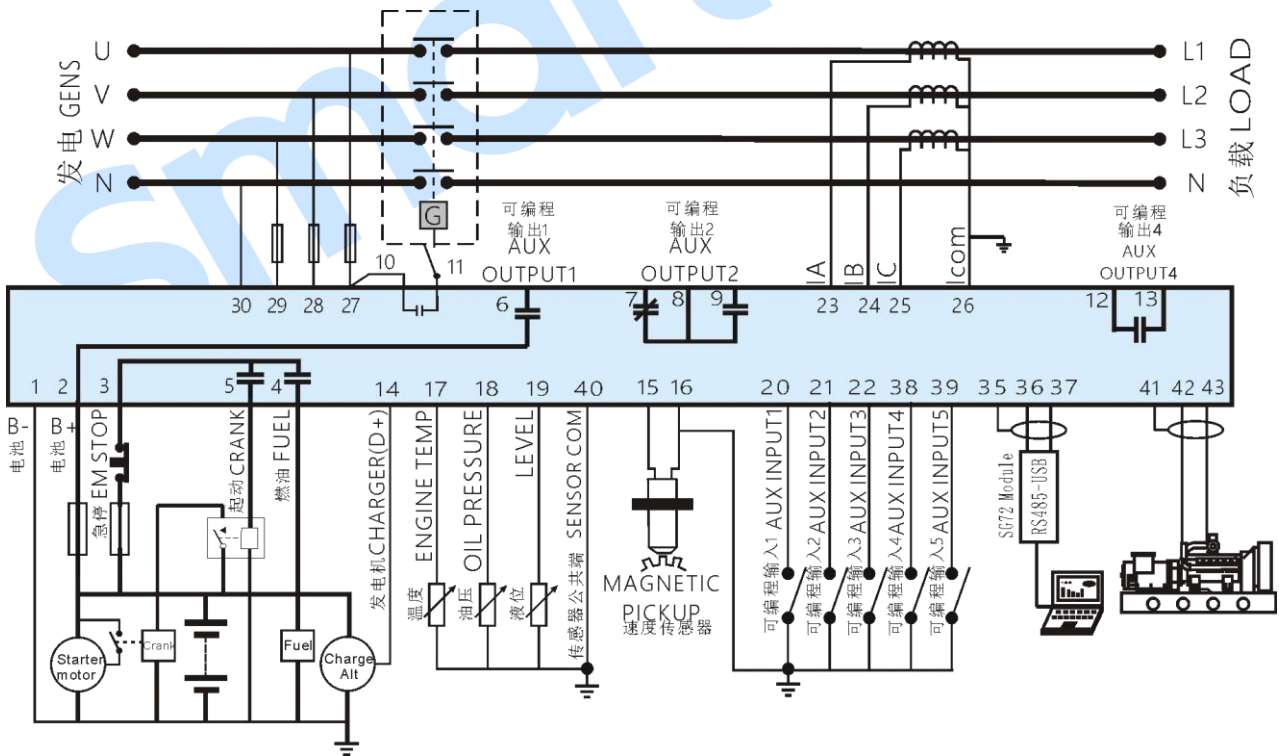
图5 HGM6110LT 典型应用图
