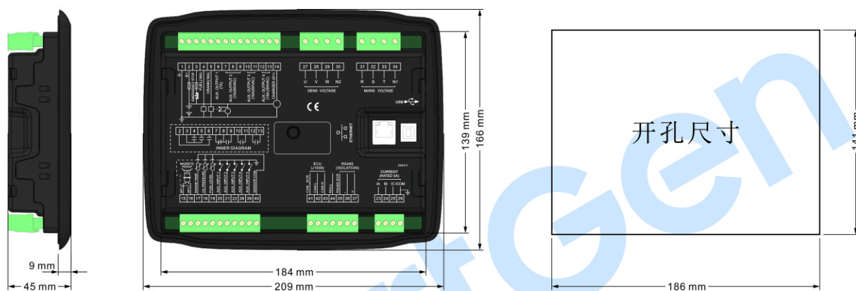
图9 外形及开孔尺寸
