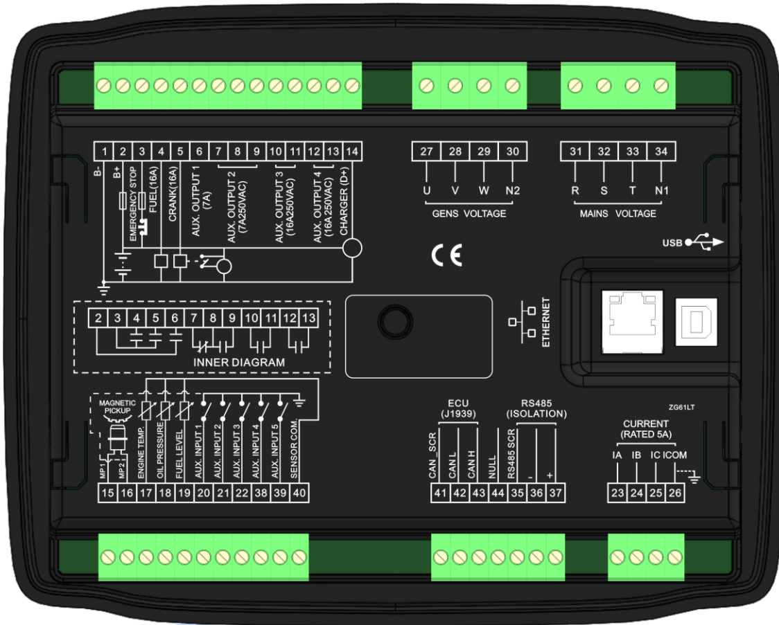
图3 控制器背面板图
