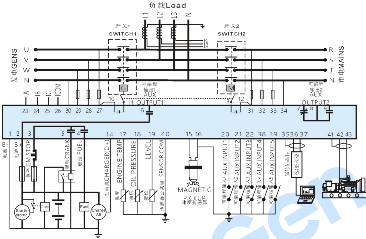
图6 HGM6120LT 典型应用图
