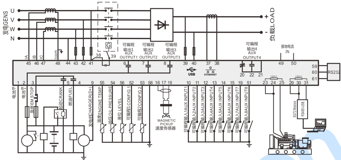
图4 HGM8110DC-1 典型应用图
