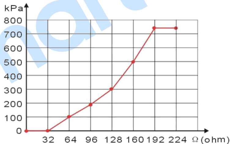
图3 曲线设置
