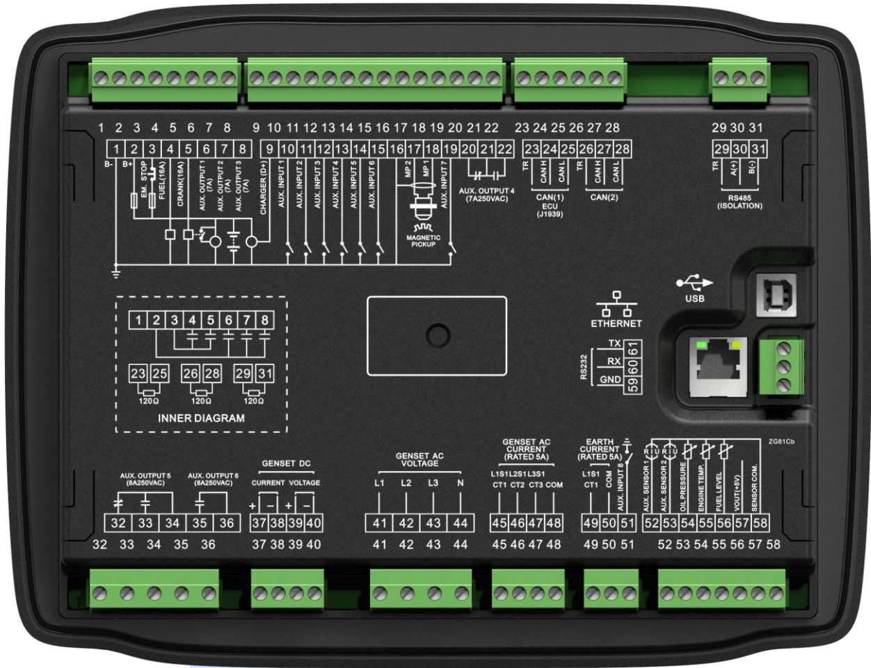
图2 控制器背面板图
