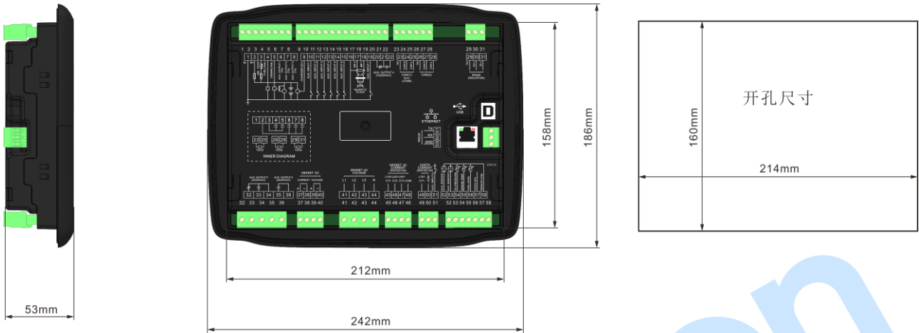
图6 外形及开孔尺寸
