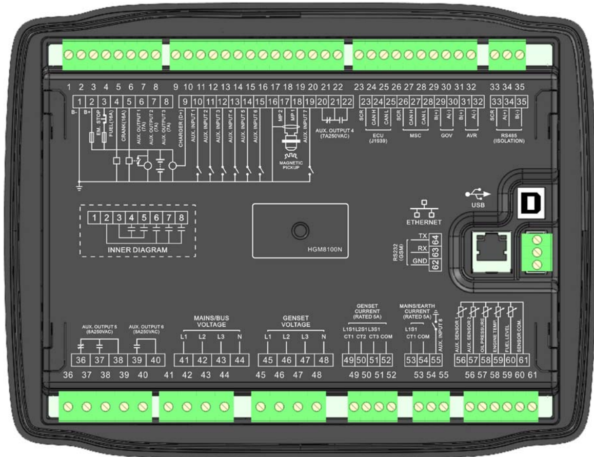
图1 控制器背面板图
