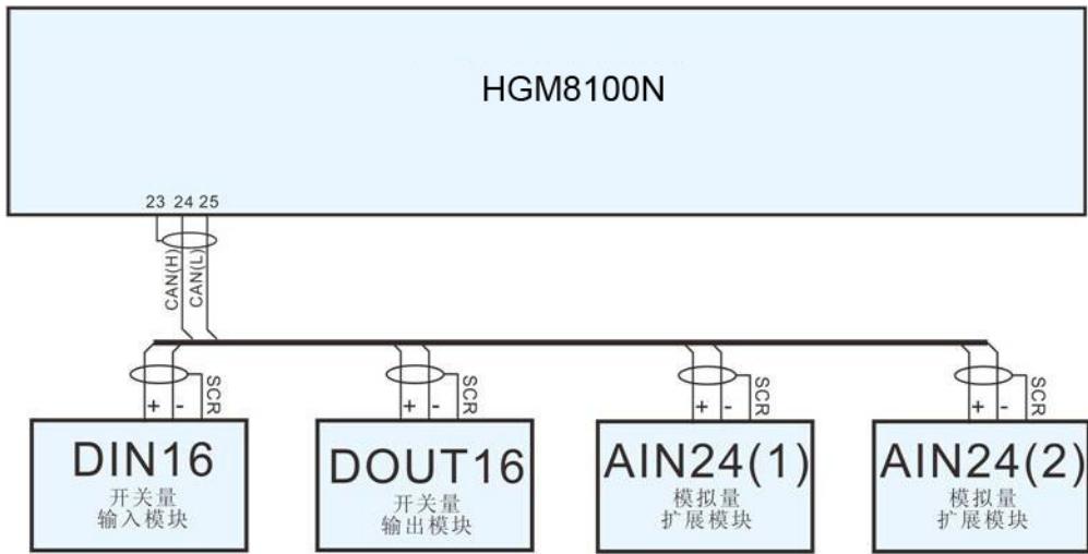
图5 HGM8100N 扩展模块典型应用图
