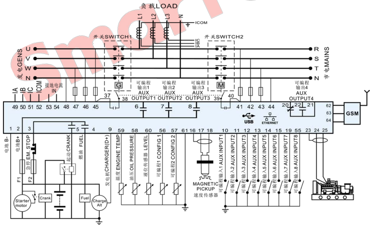
图4 HGM8120N 典型应用图
