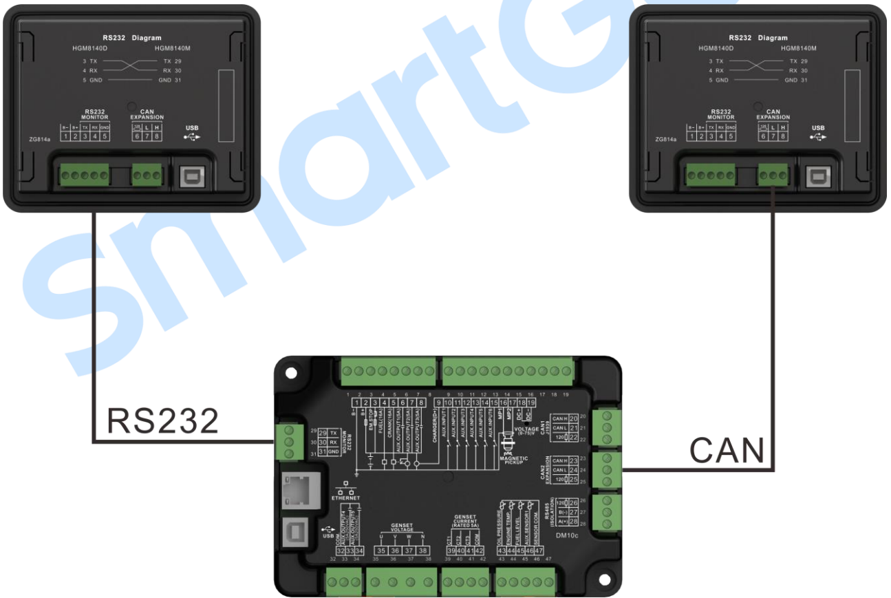
图8 HGM8140 连接示意图
