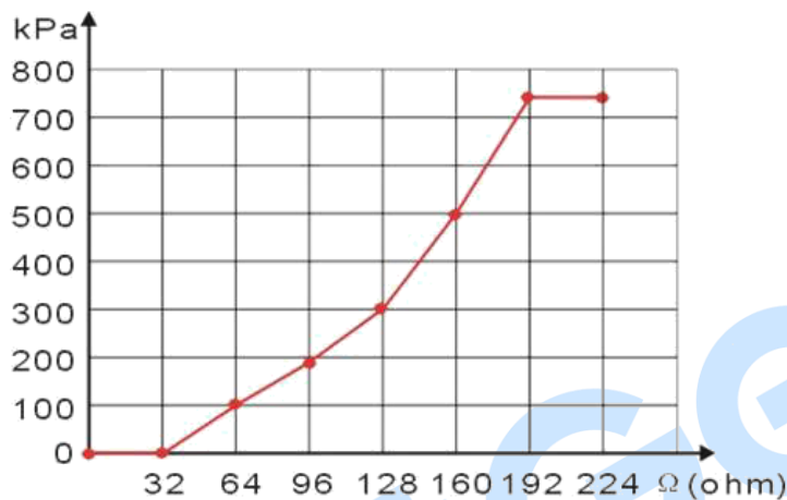
图6 压力传感器曲线
