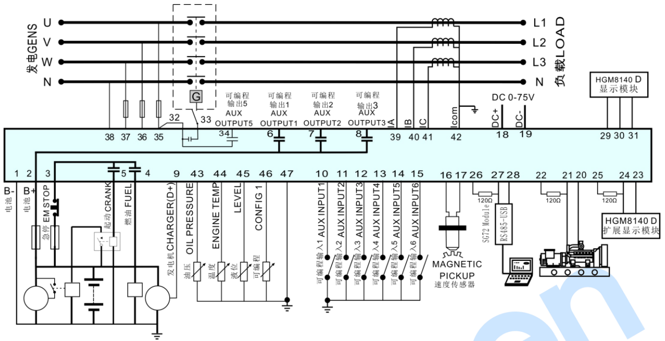
图7 HGM8140M 典型应用图
