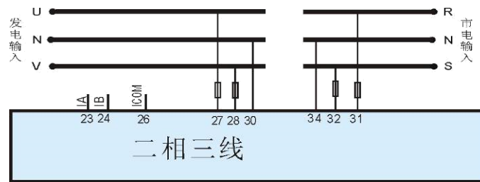
图10 二相三线连接时接线图
