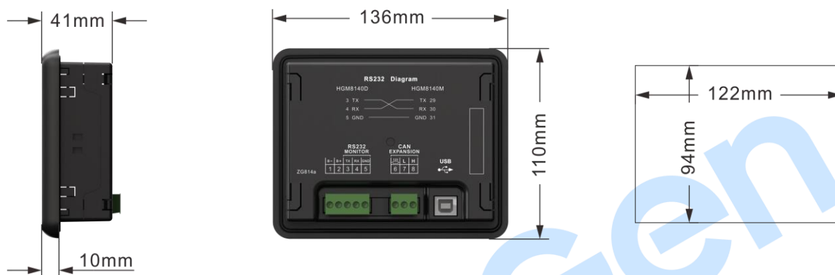
图11 HGM8140D 外形及开孔尺寸
