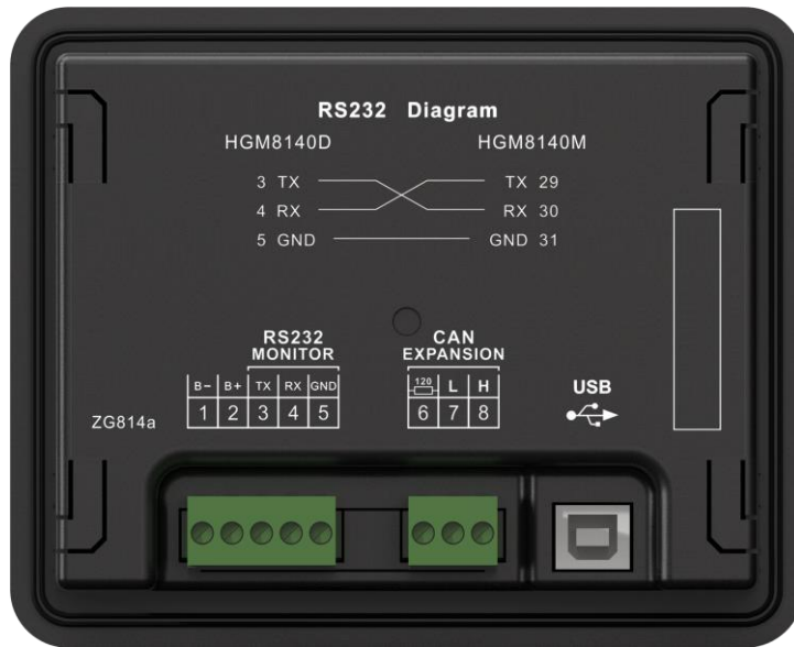
图5 HGM8140D 背部面板
