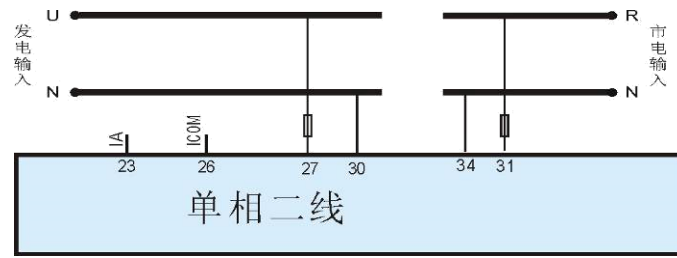
图9 单相两线接线图
