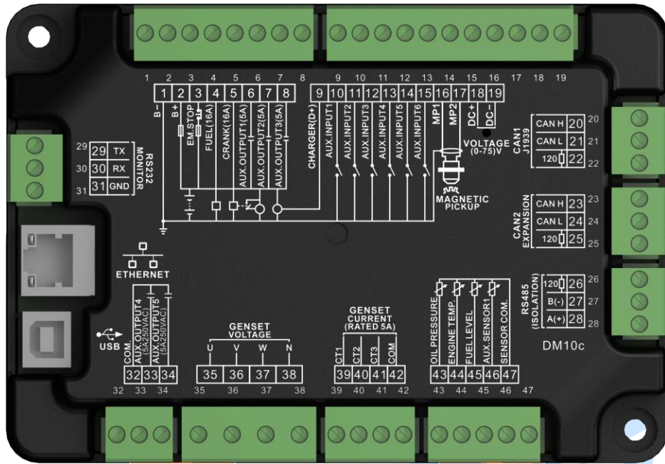
图4 HGM8140M 控制器面板图
