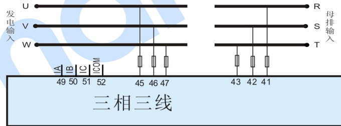
图 5 三相三线应用图
