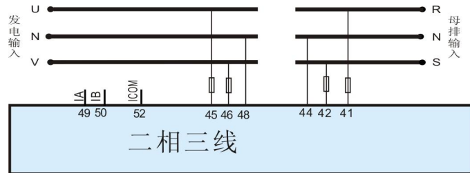
图 6 二相三线应用图
