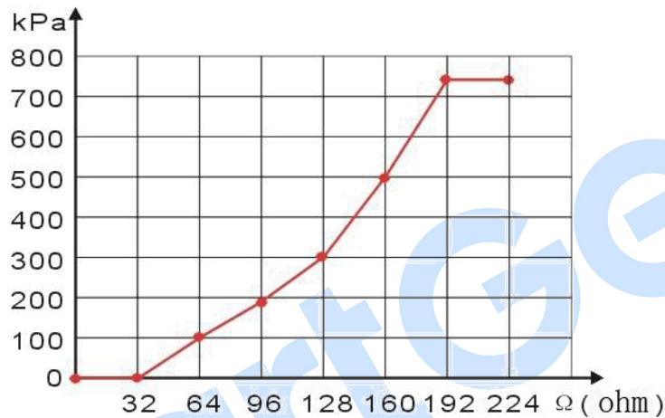
图 3 传感器曲线图
