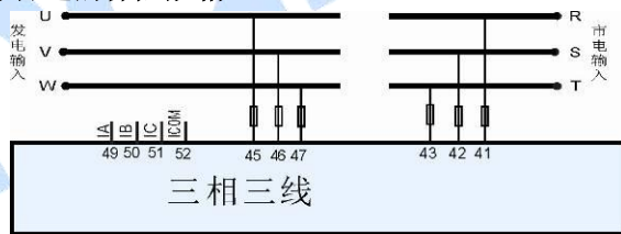
图 10 三相三线应用图
