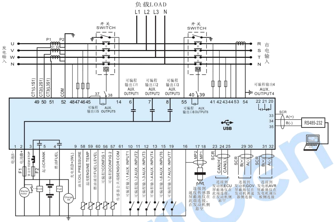
图 9 HGM9520 三相四线典型应用图
