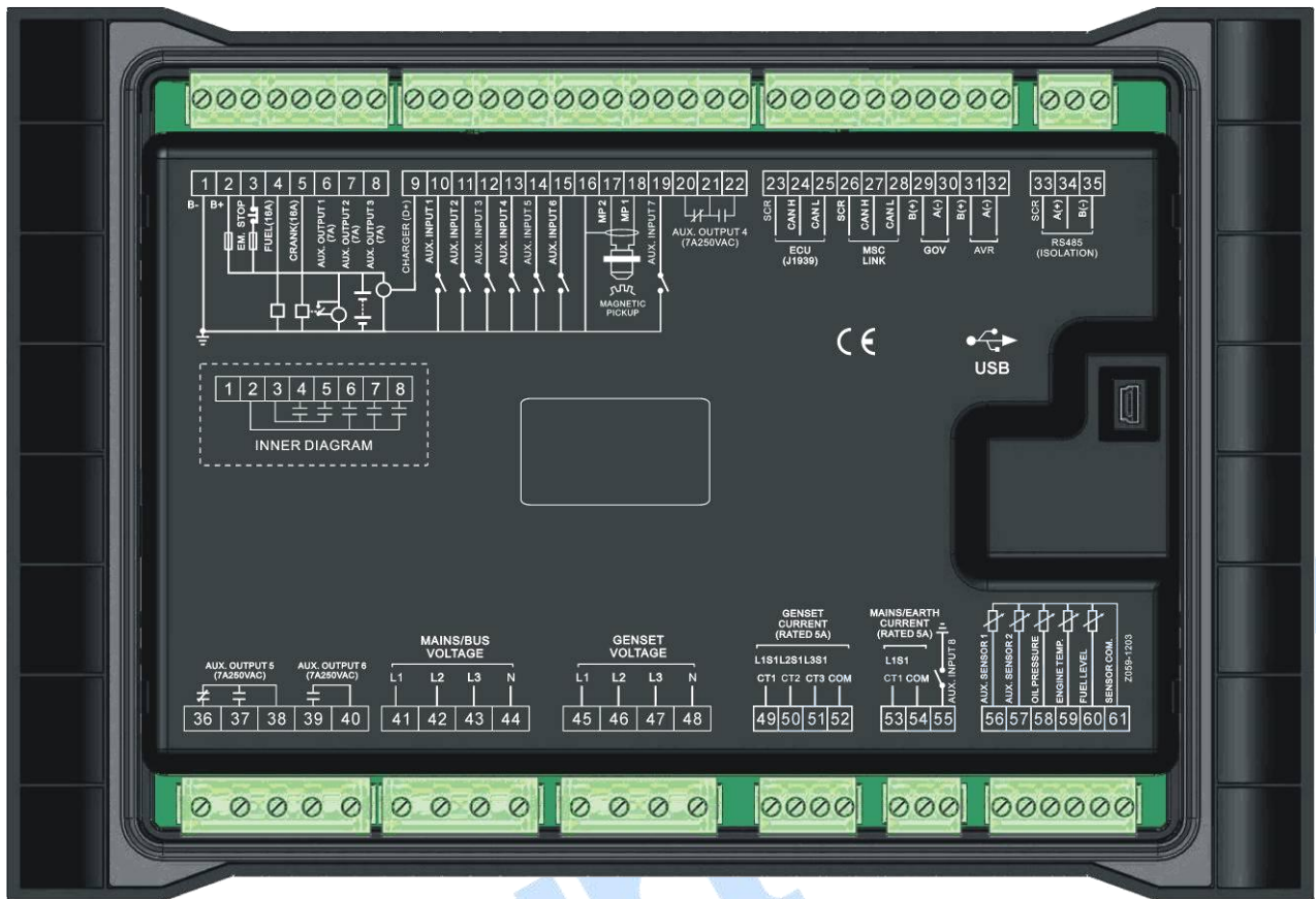
图 2 控制器背面板图
