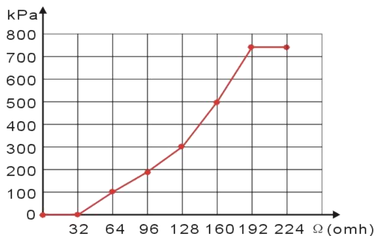
图 3 传感器曲线设置示例图
