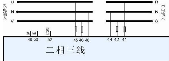
图 11 二相三线应用图
