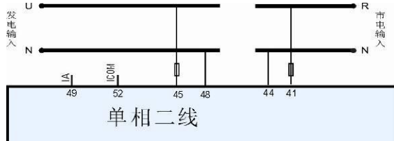
图 12 单相二线应用图
