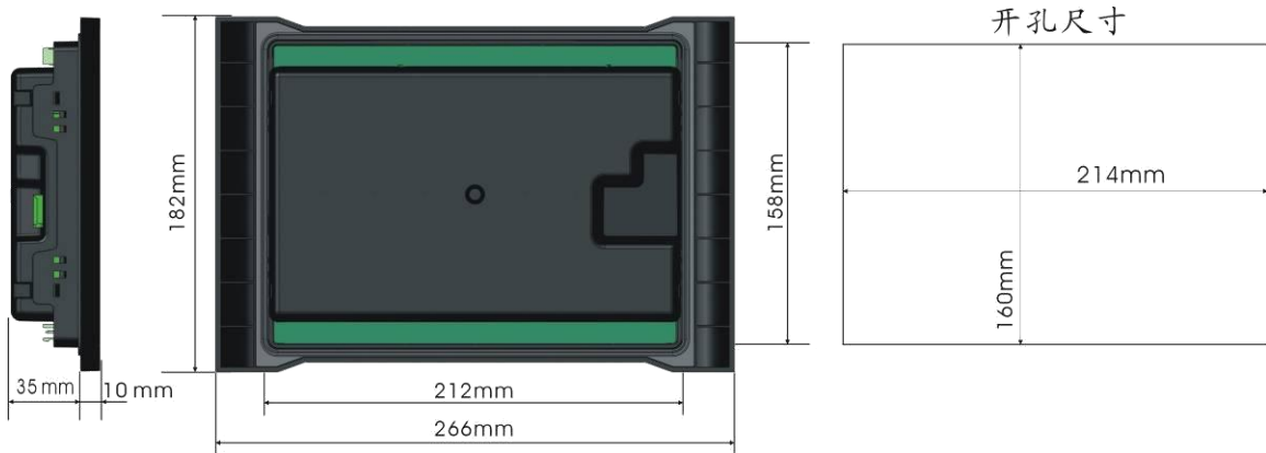
图 13 外形尺寸及面板开孔尺寸图
