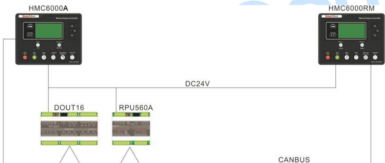
图4 HMC6000A CANBUS 通讯图
