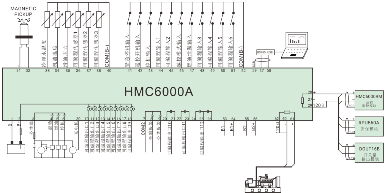
图5 HMC6000A 应用图
