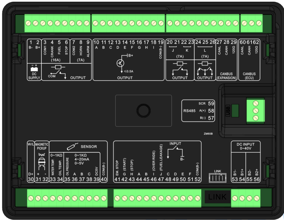
图3 HMC6000A 控制器背面板
