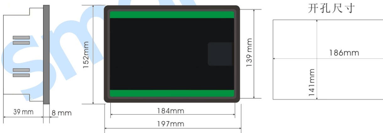
图 5 外形及开孔尺寸
