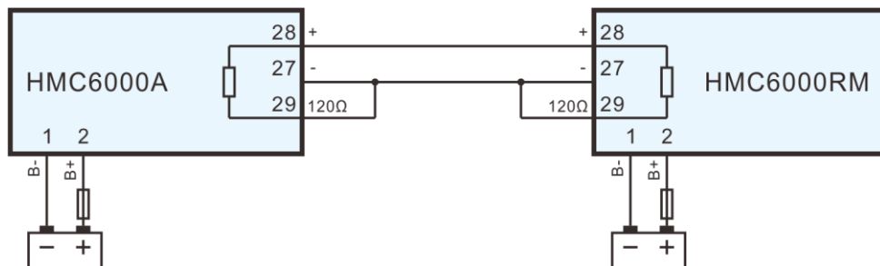
图 3 HMC6000RM 应用图
