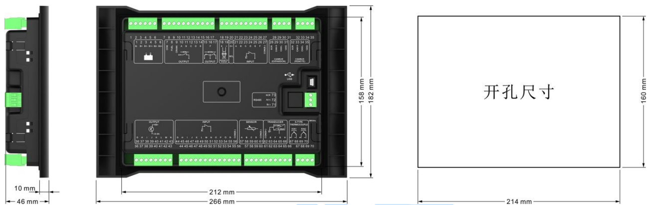
图7 安装尺寸图
