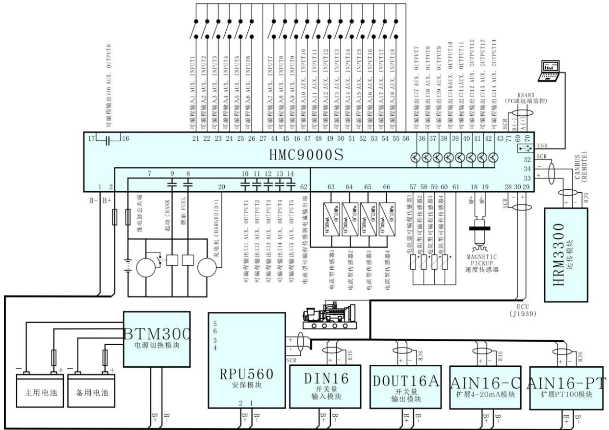
图5 HMC9000S 典型接线图
