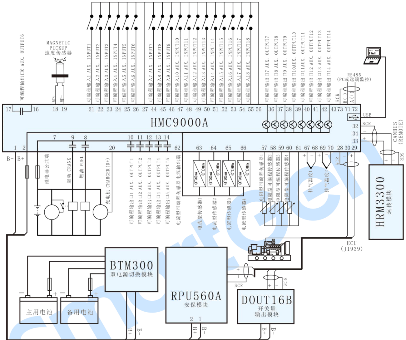
图4 HMC9000A 典型接线图
