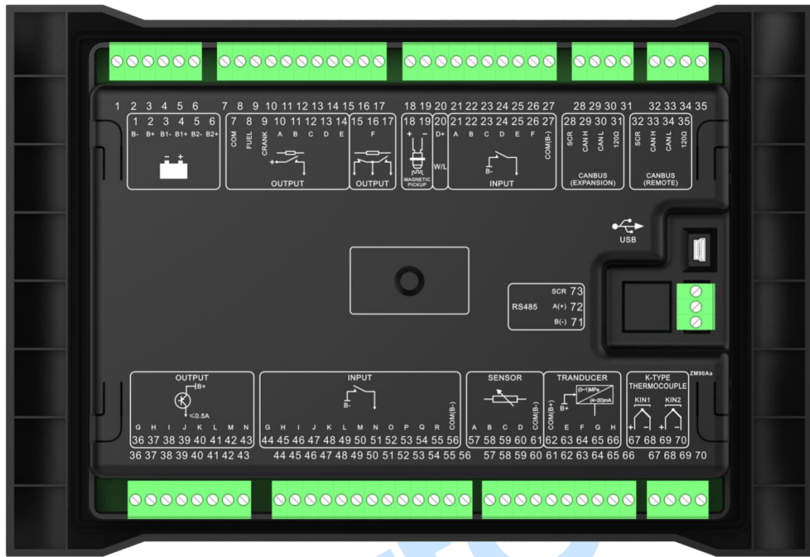
图3 HMC9000A/S 控制器背面板
