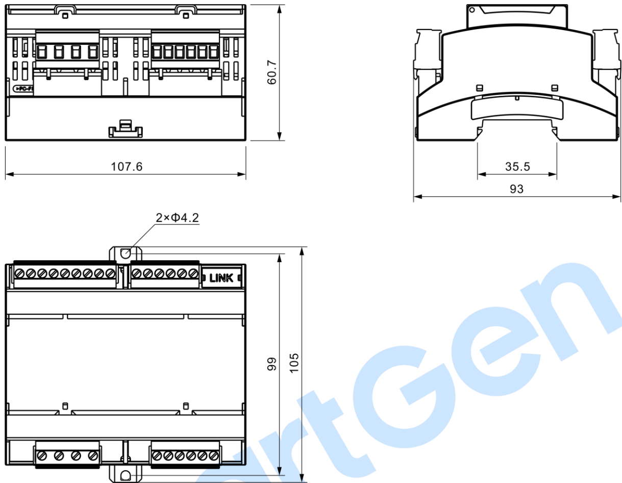
图4 外形及开孔尺寸
