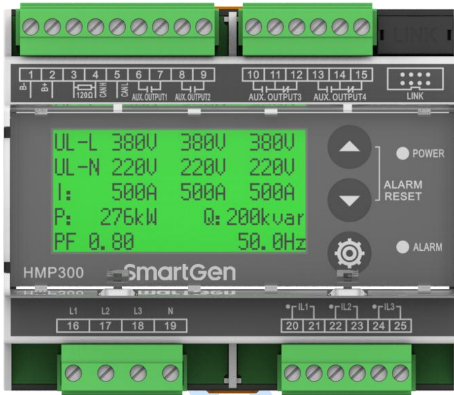
图1 模块面板图
