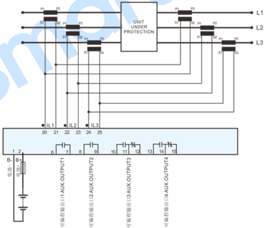
图3 差动保护应用图
