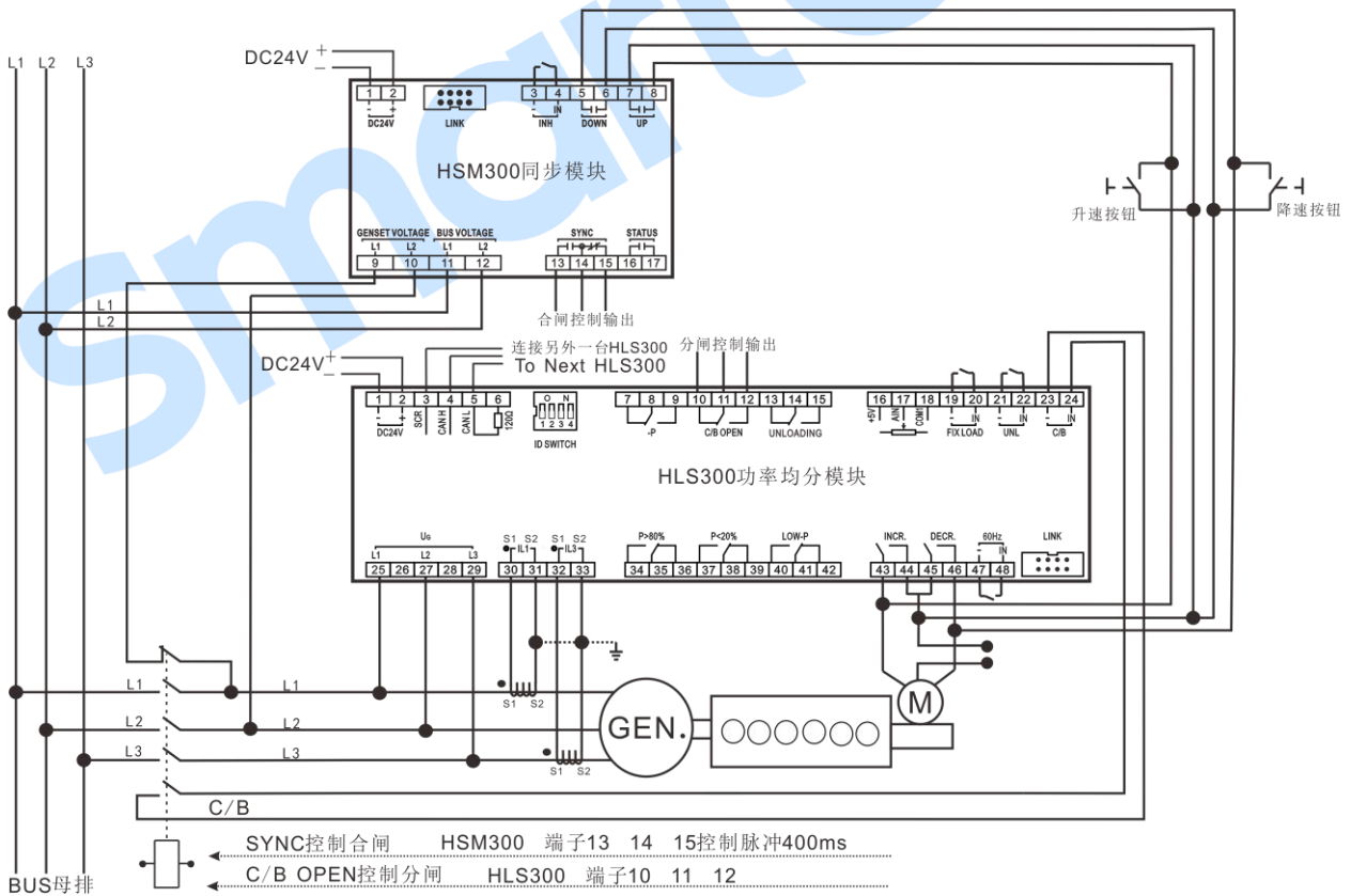
图5 HSM300-HLS300 三相三线典型应用图
