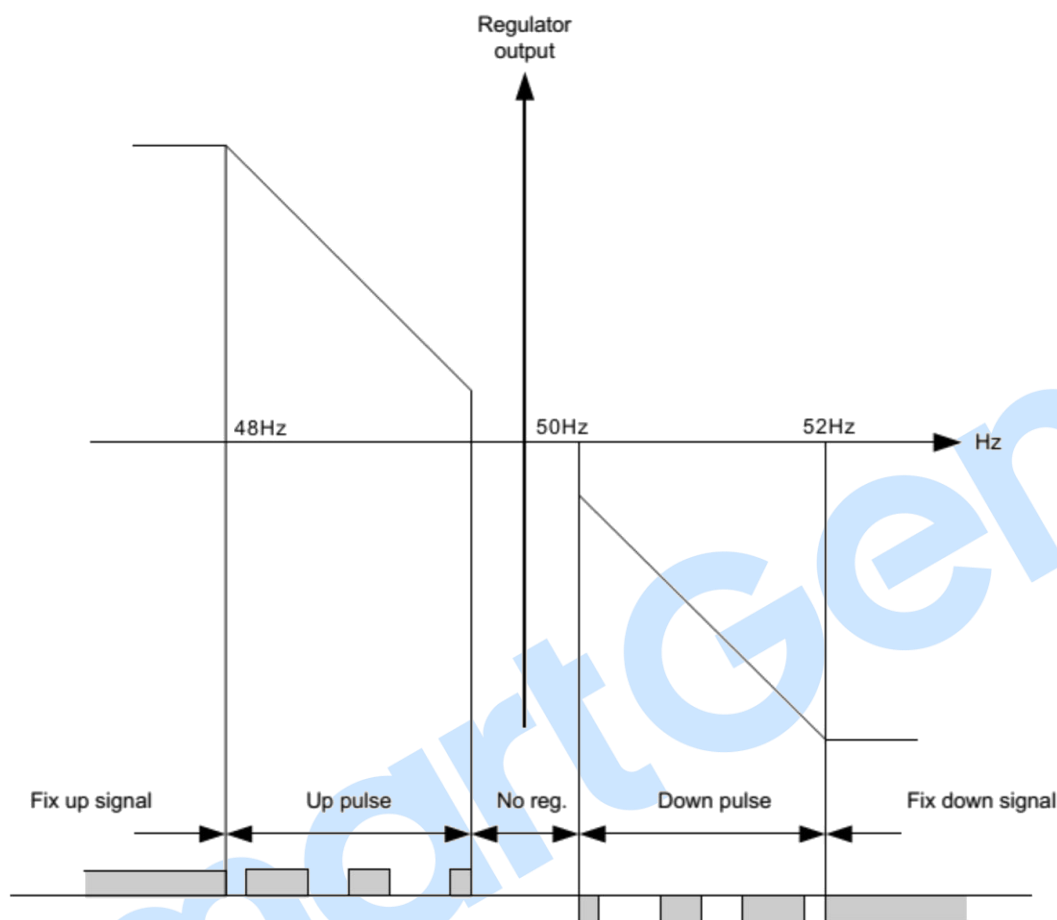
图3 升/降速继电器工作原理图
