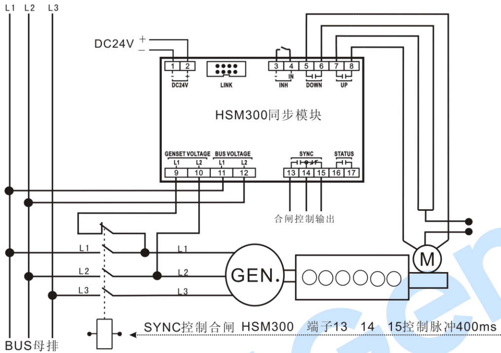
图4 HSM300 三相三线典型应用图
