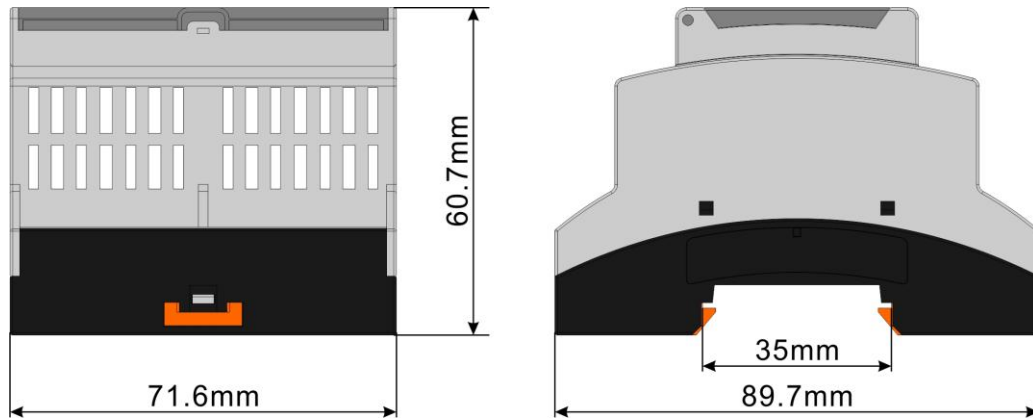
图6 外形尺寸图
