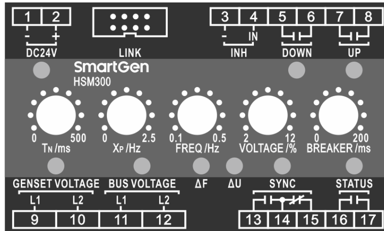
图1 面膜图
